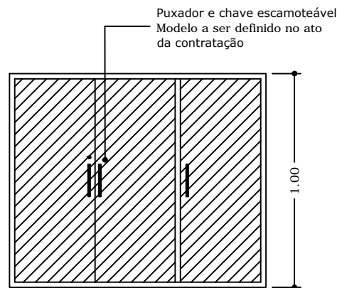
Elevação
