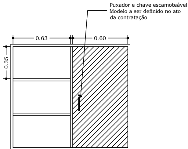
Elevação
