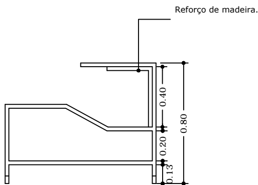
Elevação
