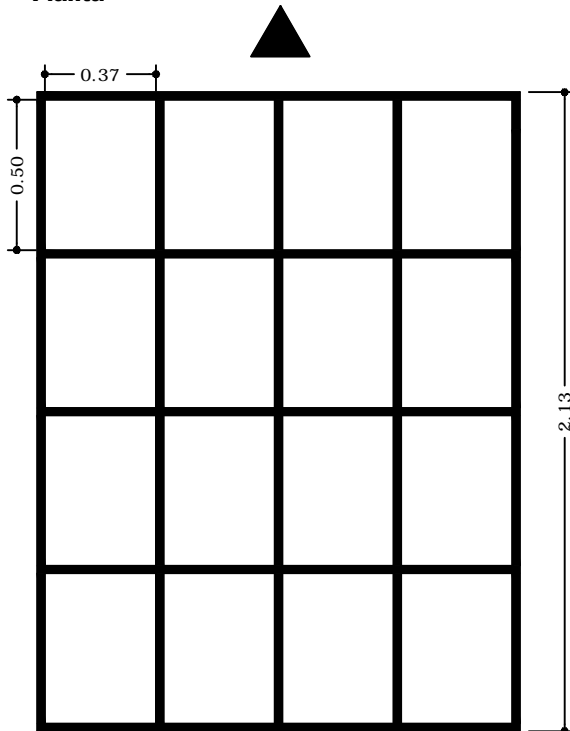
Elevação
