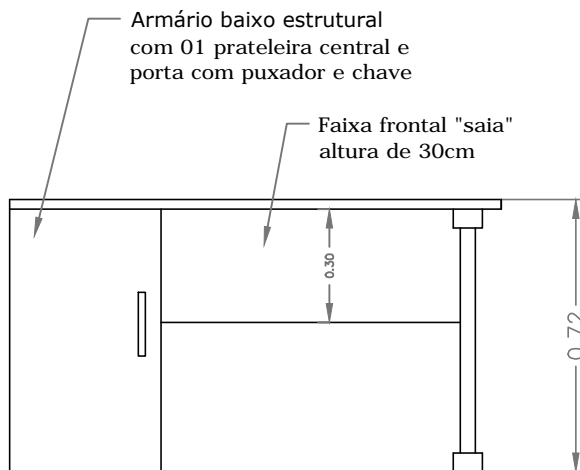
Elevação
