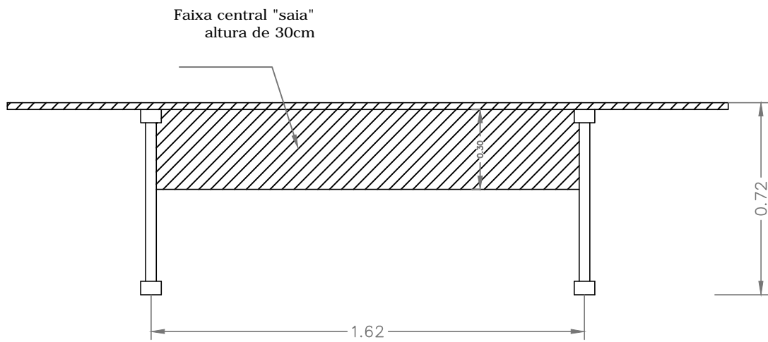
Elevação
