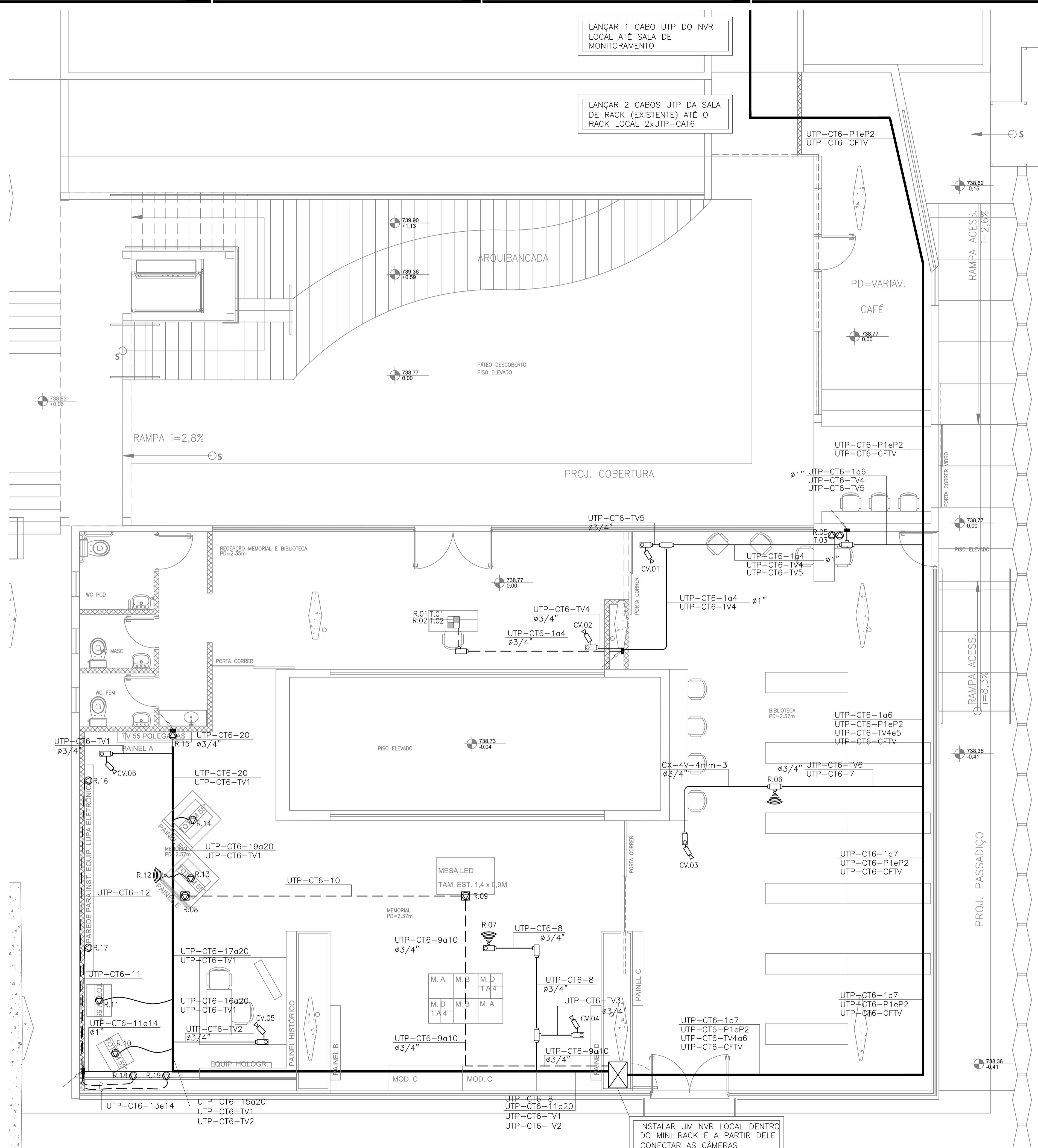
PLANTA BAIXA DE DISTRIBUIÇÃO DE PONTOS DE REDE, TELEFONIA, WI-FI E CÂMERAS DE MONITORAMENTO. ESCALA 1:50
