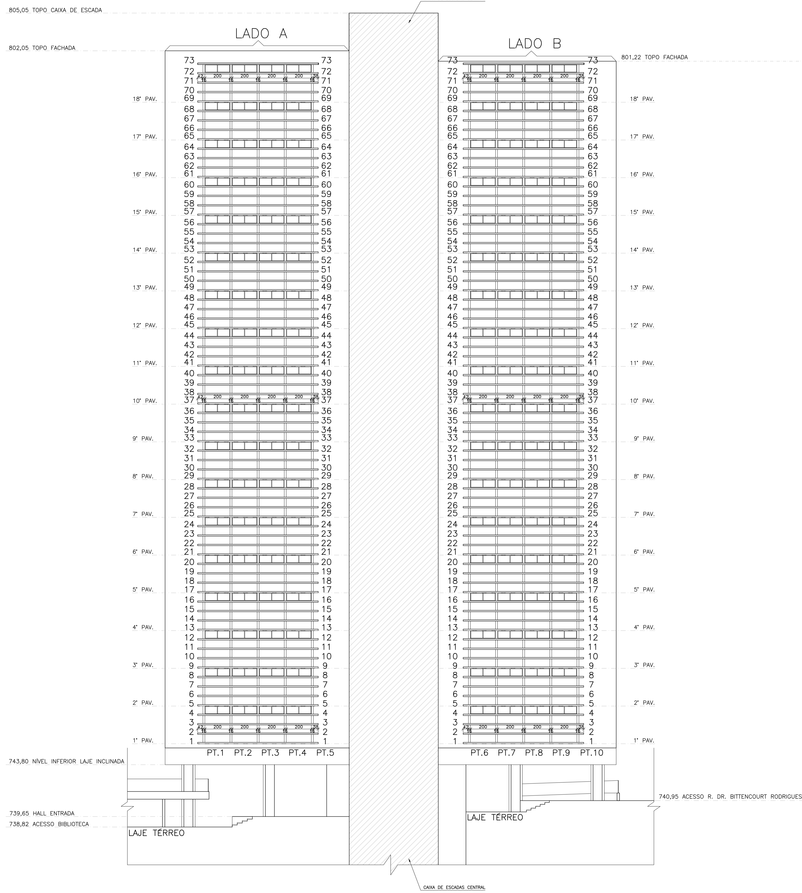
ELEVACÃO DA FACHADA DOS BRISES EDIFÍCIO SEDE 1:150
