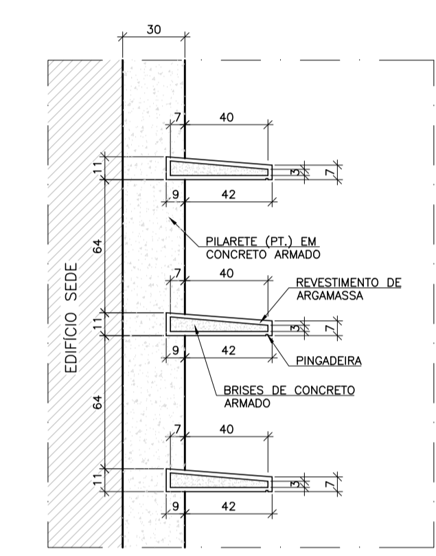
CORTE TÍPICO DOS BRISES EDIFÍCIO SEDE 1:25
