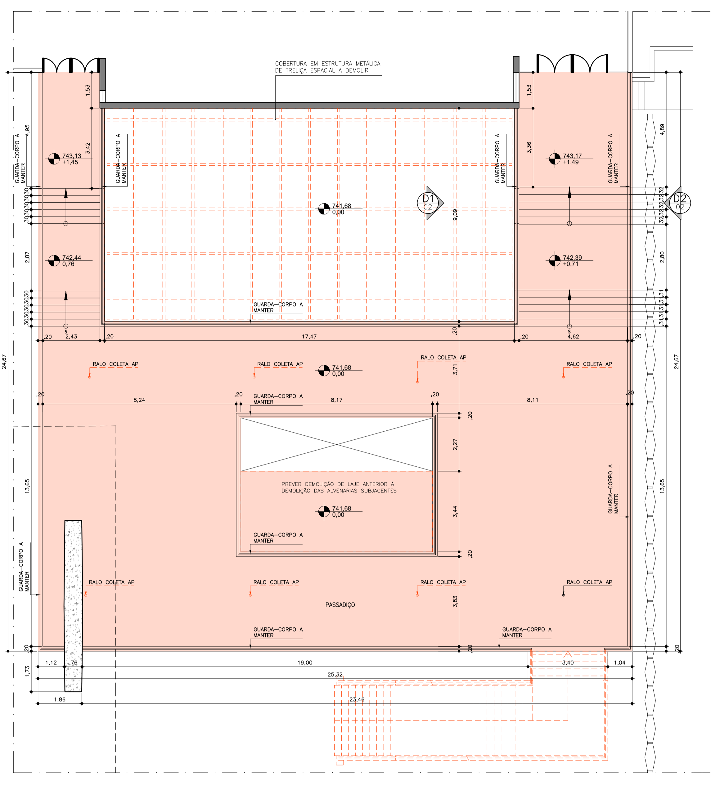
PLANTA PASSADIÇO - A DEMOLIR ESCALA 1:100
