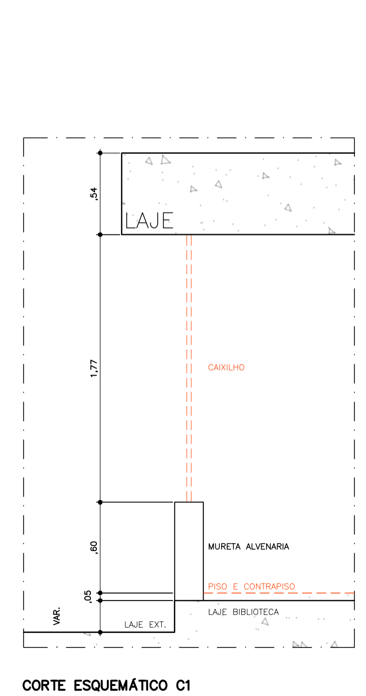
CORTE ESQUEMÁTICO C1 ESCALA 1:25
