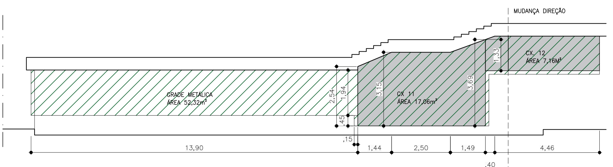
ELEVÇÃO ESQUEMÁTICA D2 ESCALA 1:100
