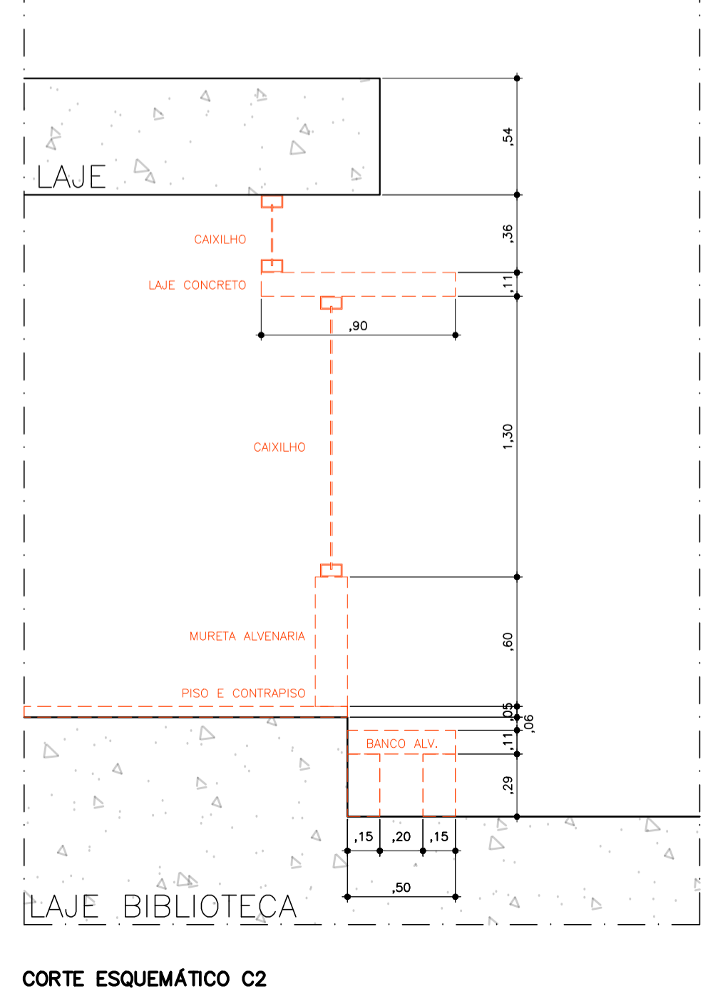
CORTE ESQUEMÁTICO C2 ESCALA 1:25
