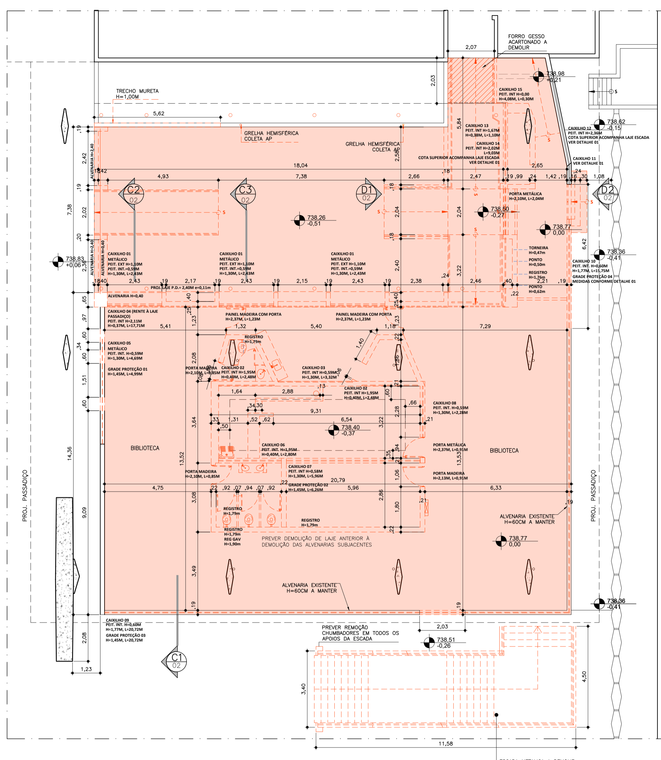
PLANTA TÉRREO - A DEMOLIR ESCALA 1:100
