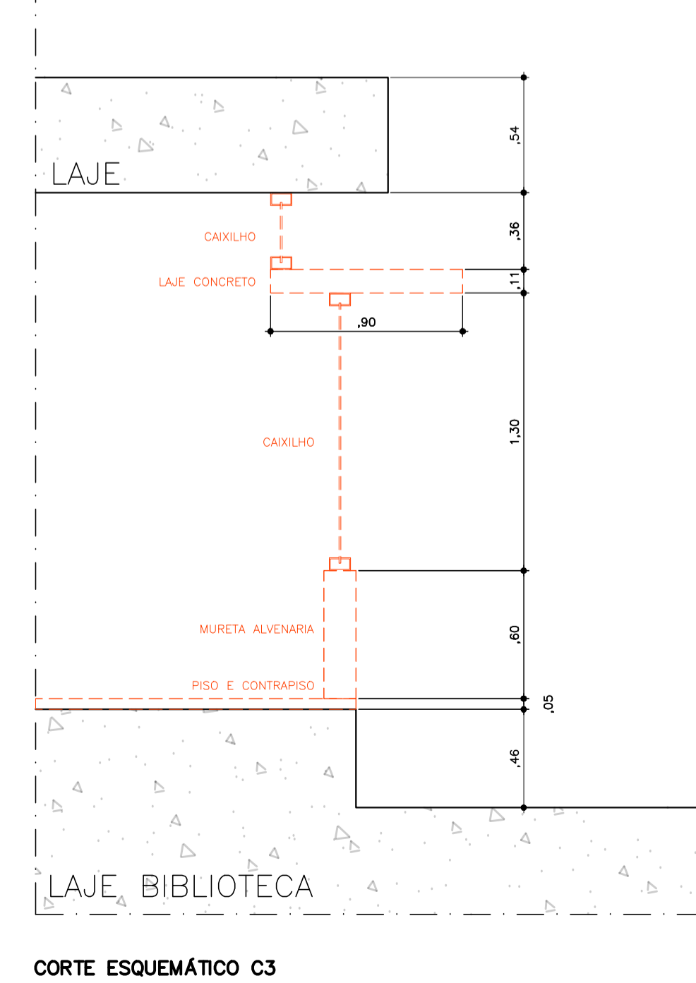
CORTE ESQUEMÁTICO C3 ESCALA 1:25
