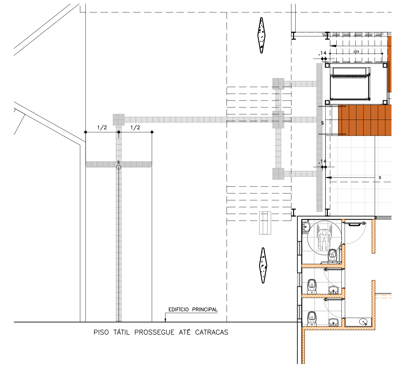
PLANTA – DETALHE PISO TÁTIL IMPLANTAÇÃO ESCALA 1:100
