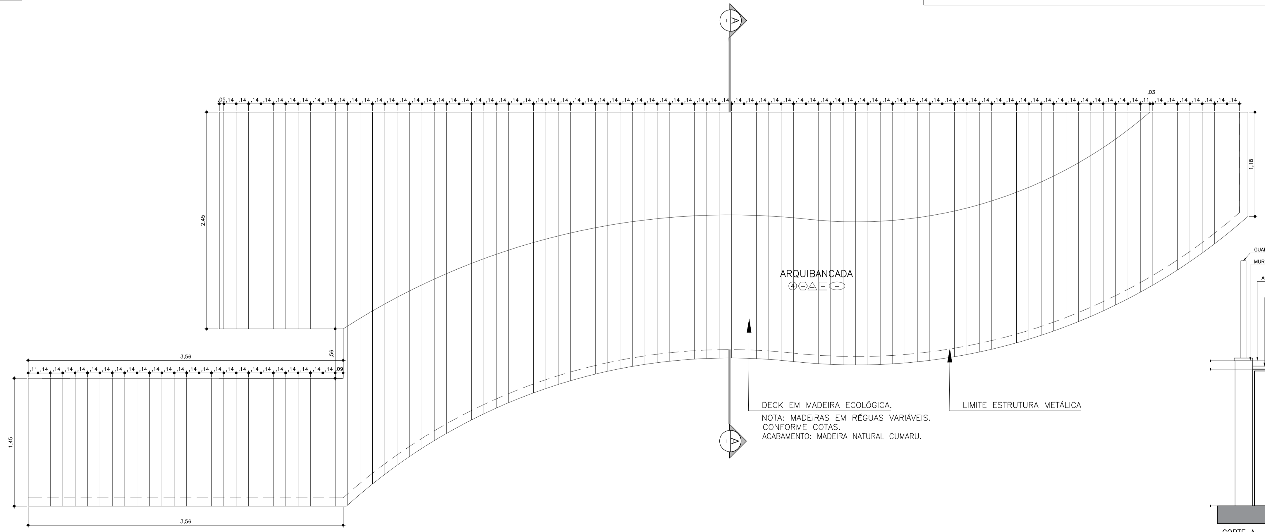
PLANTA DECK ESCALA 1:25
