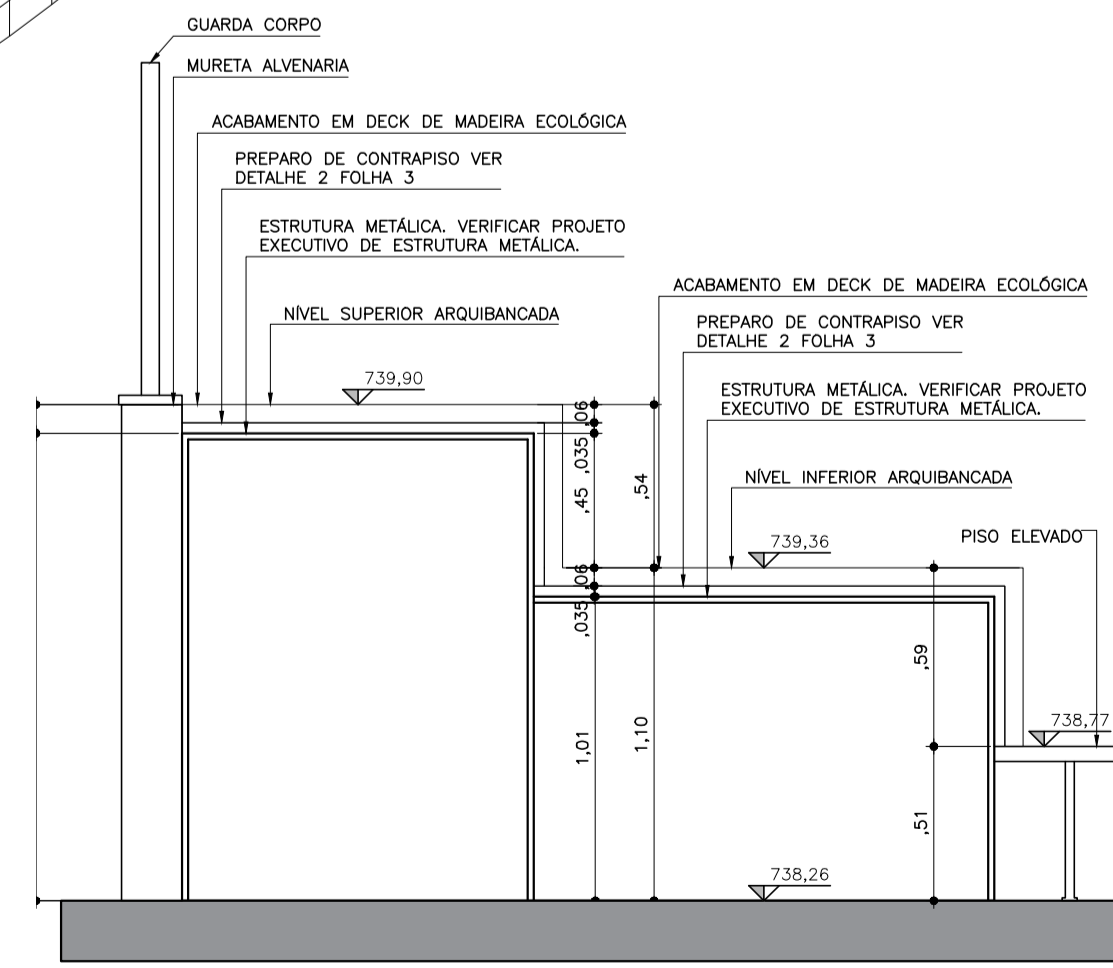
CORTE A ESCALA 1:25
