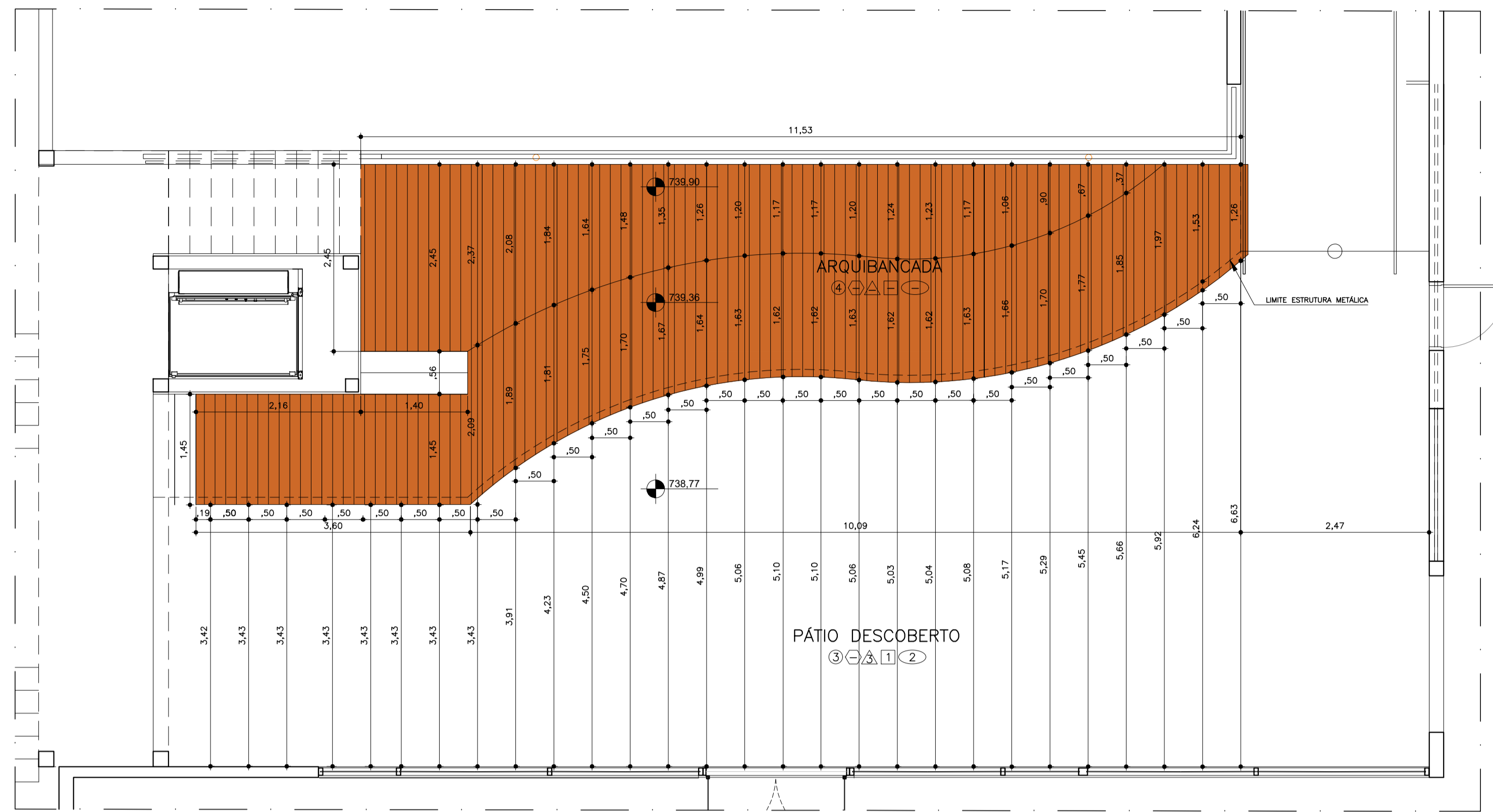
PLANTA ARQUIBANCADA – LOCAÇÃO ESCALA 1:50
