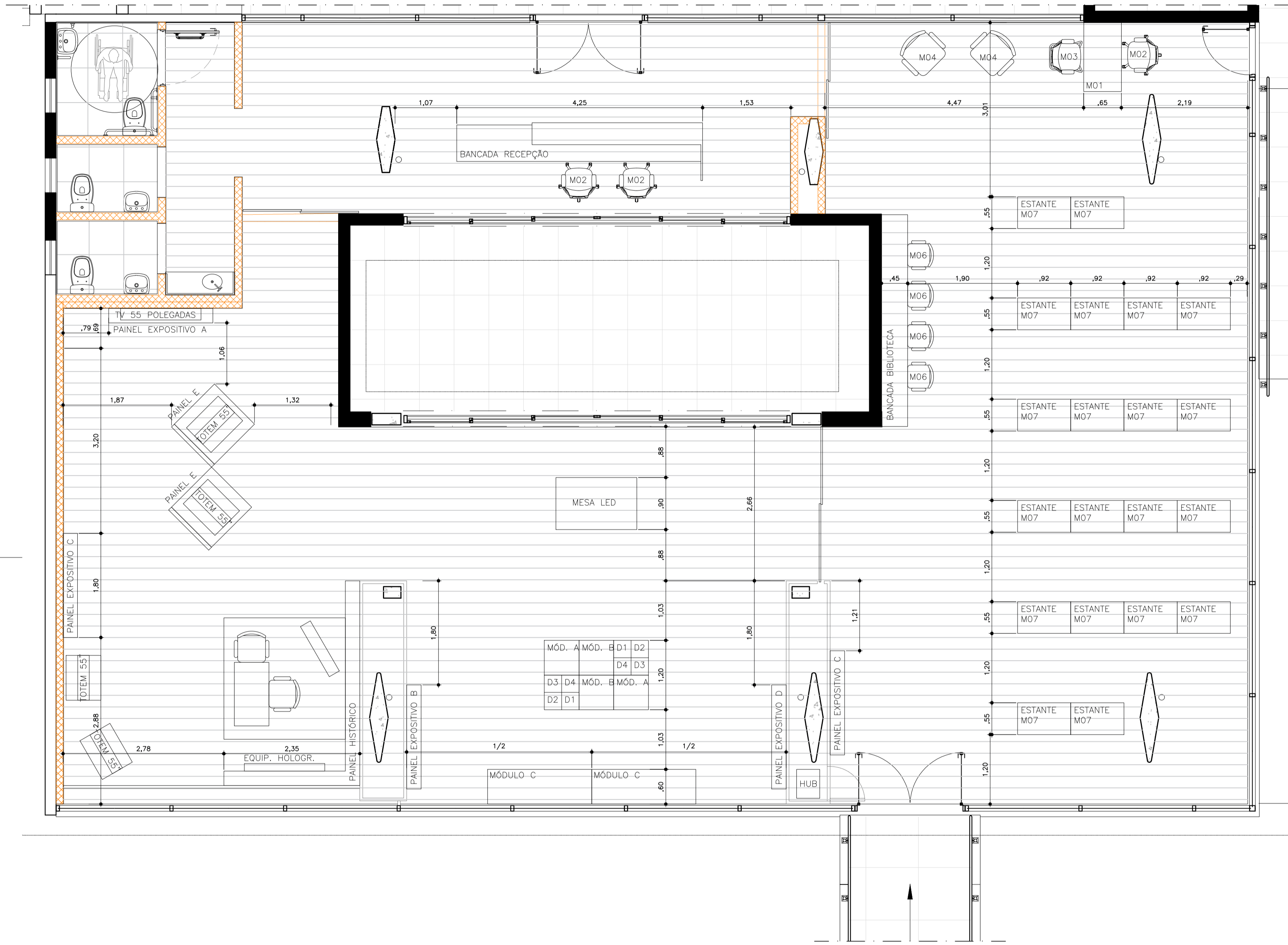
PLANTA DE LAYOUT - DISPOSIÇÃO MOBILIÁRIO SUGERIDO E PEÇAS DE MARCENARIA ESCALA 1:50
