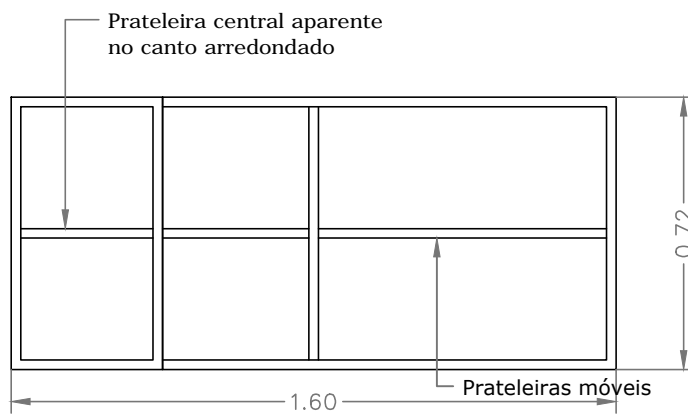
Elevação
