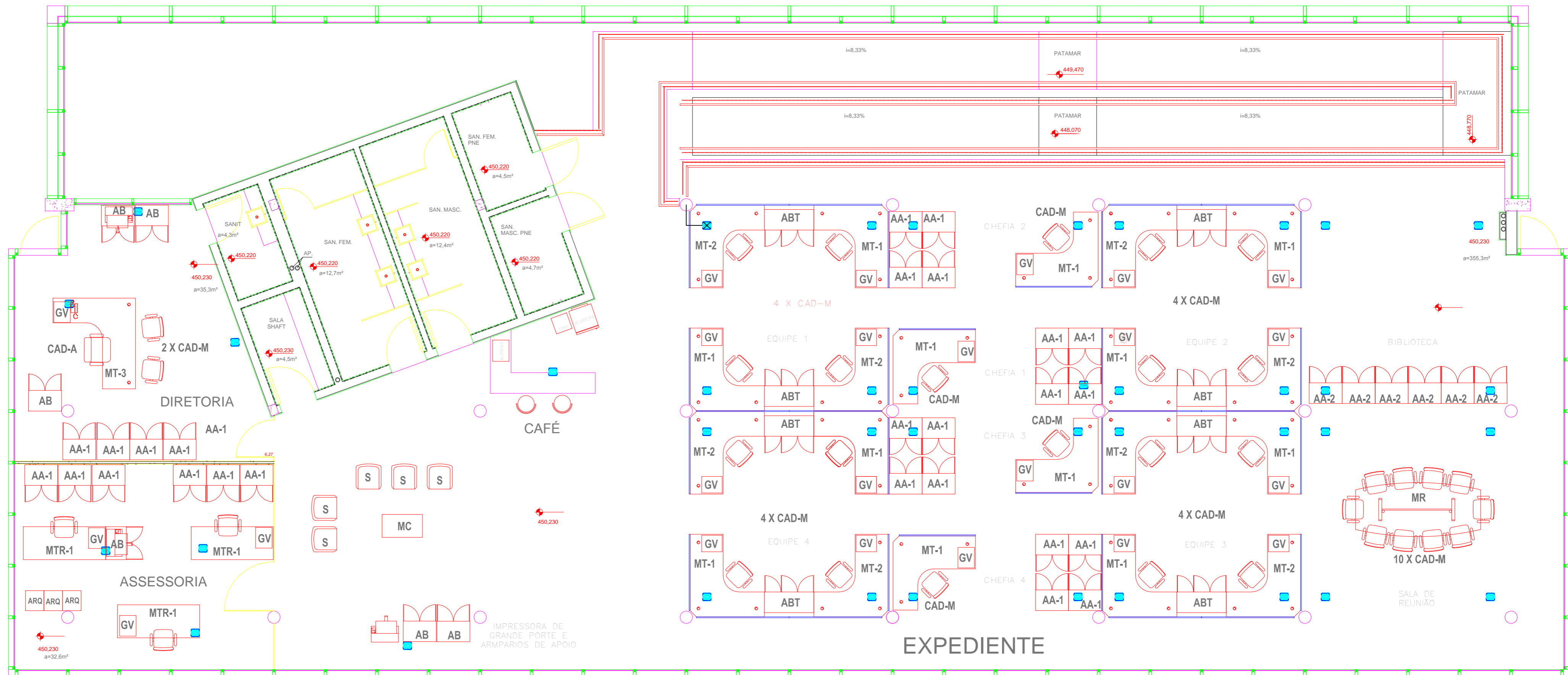
LAYOUT MOBILIÁRIO UR 18 ADAMANTINA PAVIMENTO SUPERIOR
