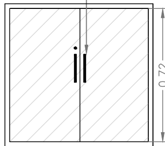
Elevação
