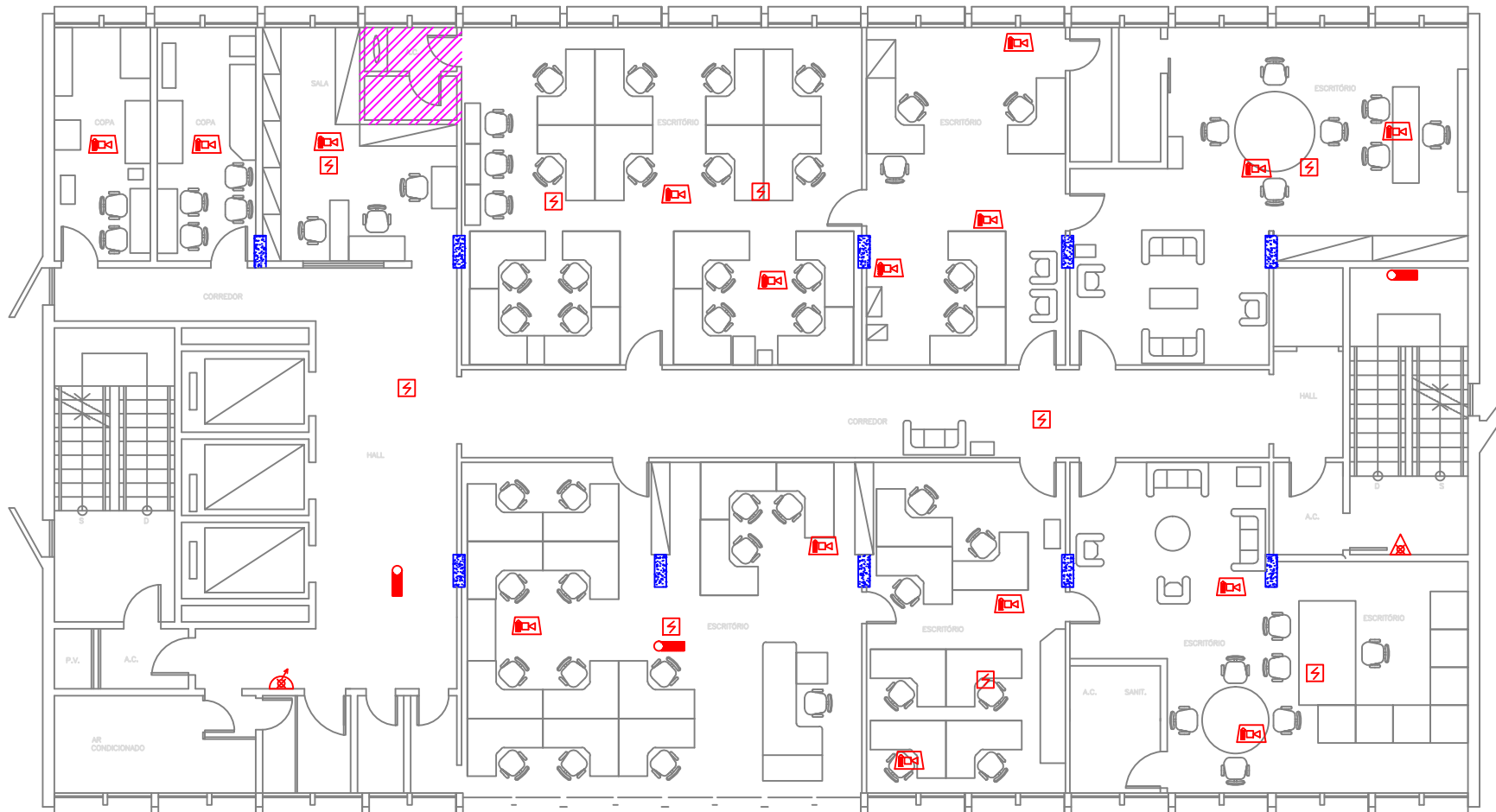
PLANTA DO 5º PAVIMENTO – ANEXO I ESC.: 1:100
