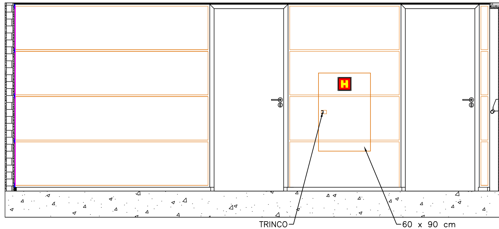
CORTE GG
