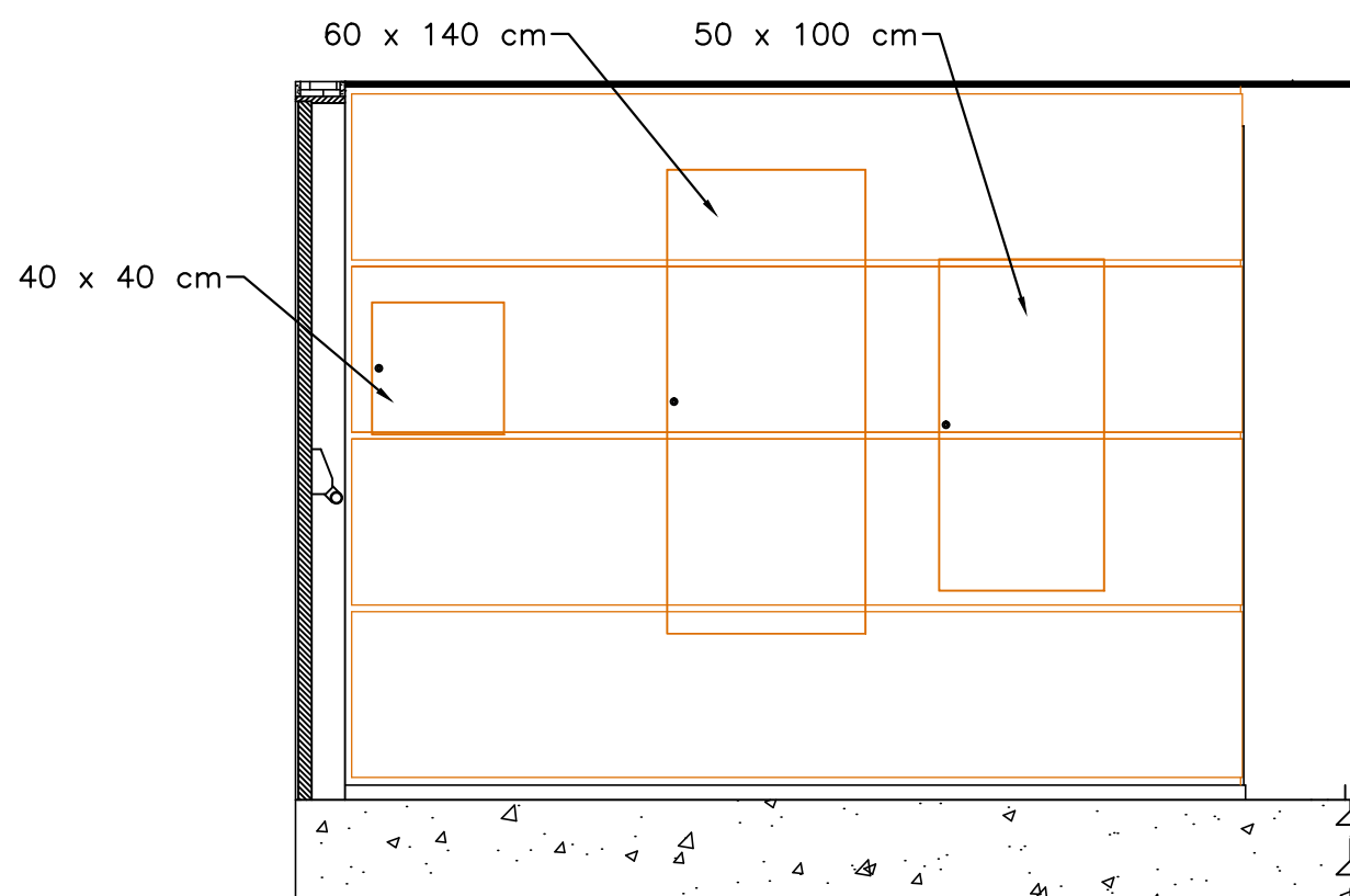
CORTE FF
