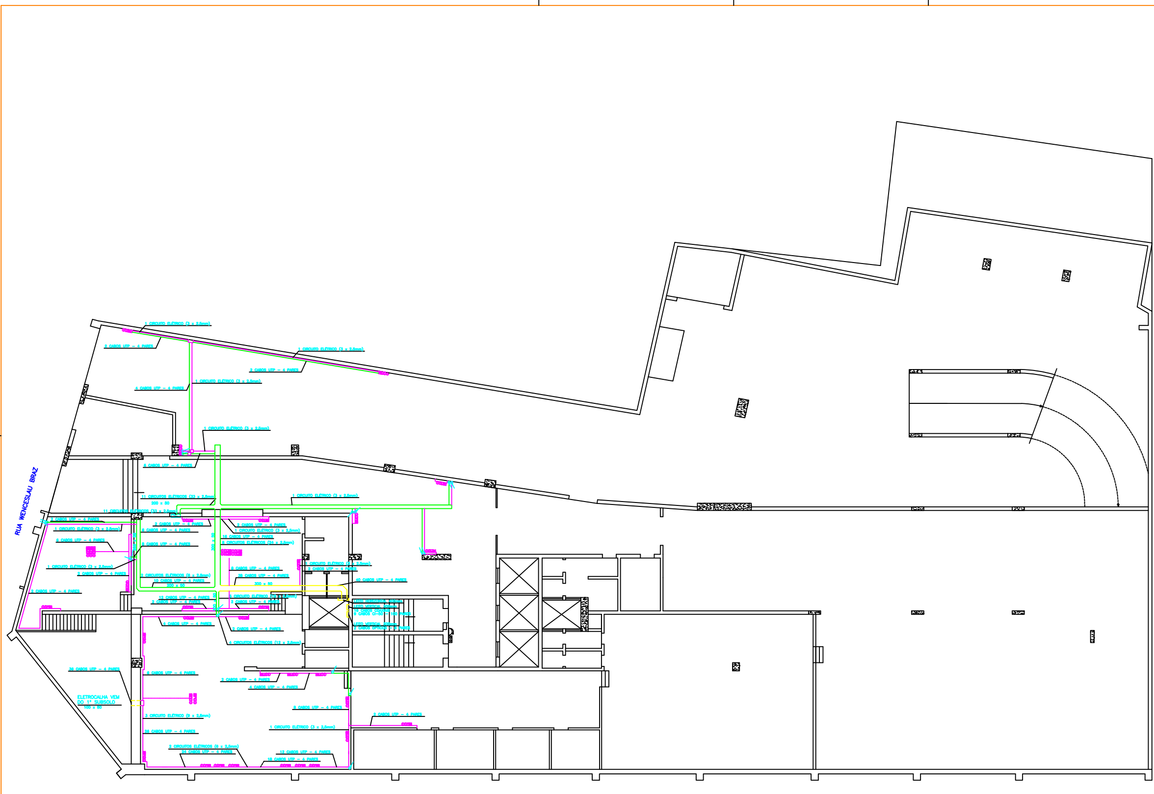
PLANTA - TÉRREO ESC. 1/75
