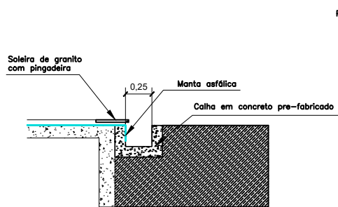
DETALHE CANALETA – PERÍMETRO A
