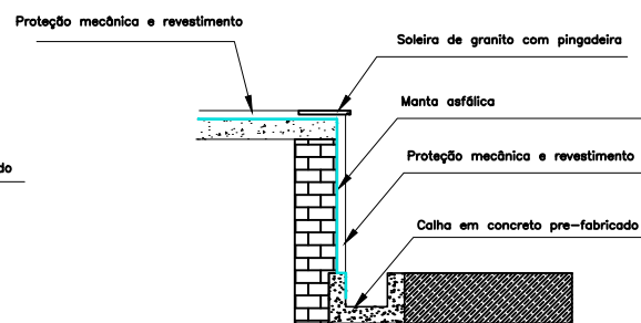
DETALHE CANALETA – PERÍMETRO B
