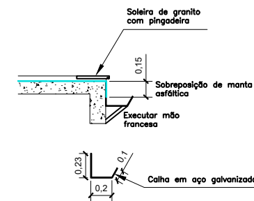
DETALHE CANALETA – PERÍMETRO C
