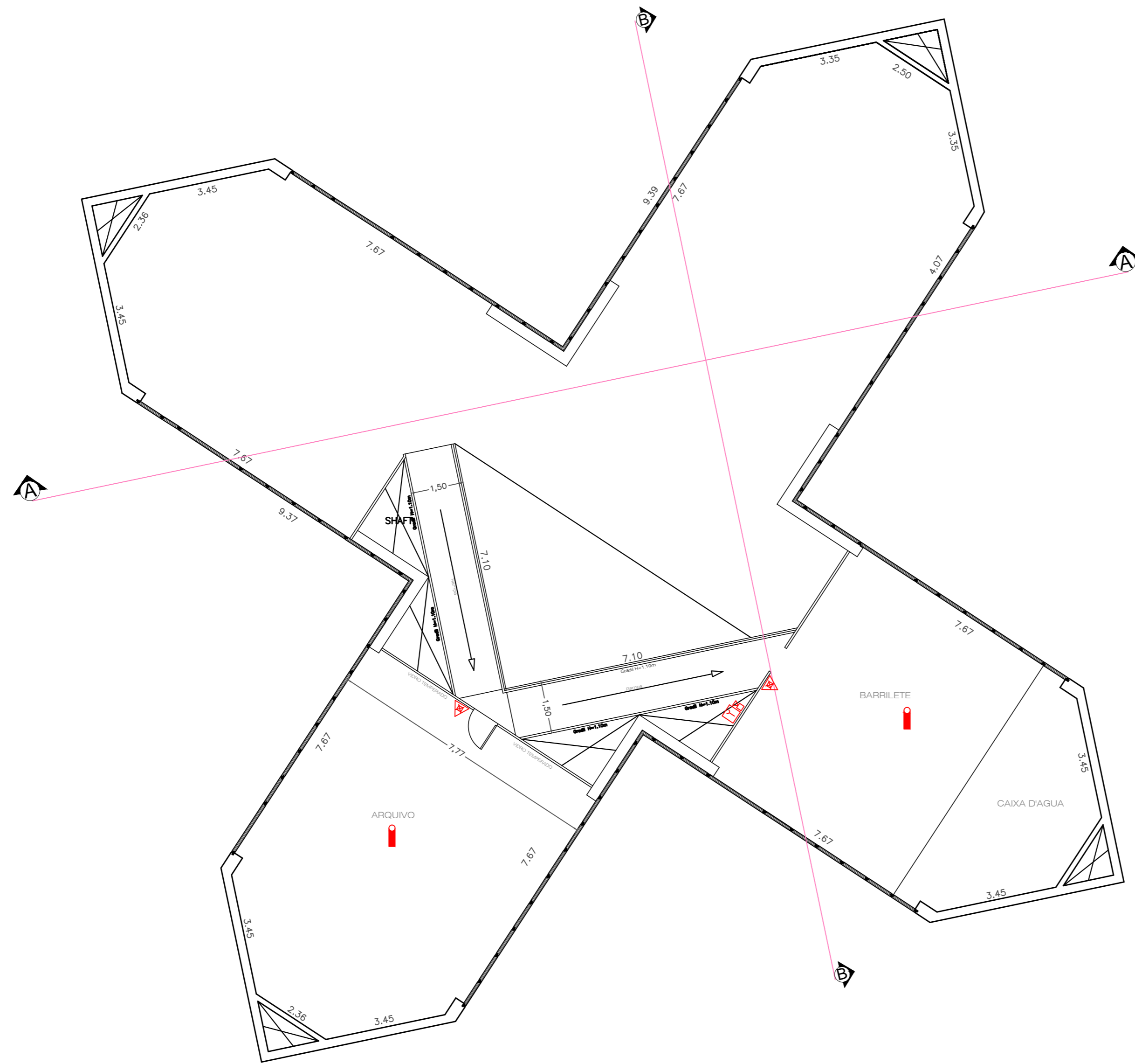
PLANTA BAIXA BARRILETE/ CAIXA D'AGUA ESCALA 1:100
