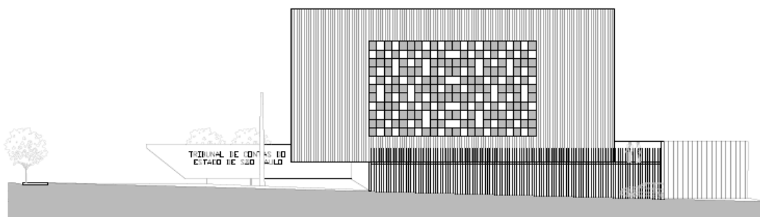
02 FACHADA 02 1/200
