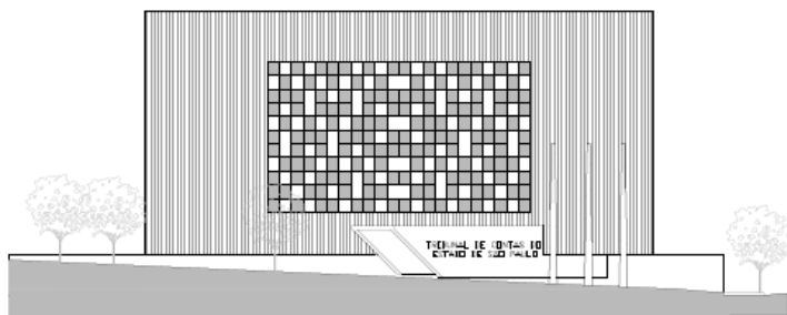
01 FACHADA 01 1/200
