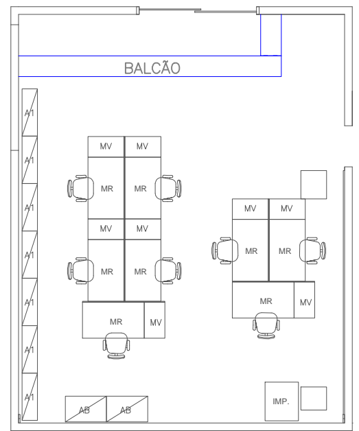
PLANTA BAIXA DA SALA ONDE SERÁ INSTALADO O BALCÃO
