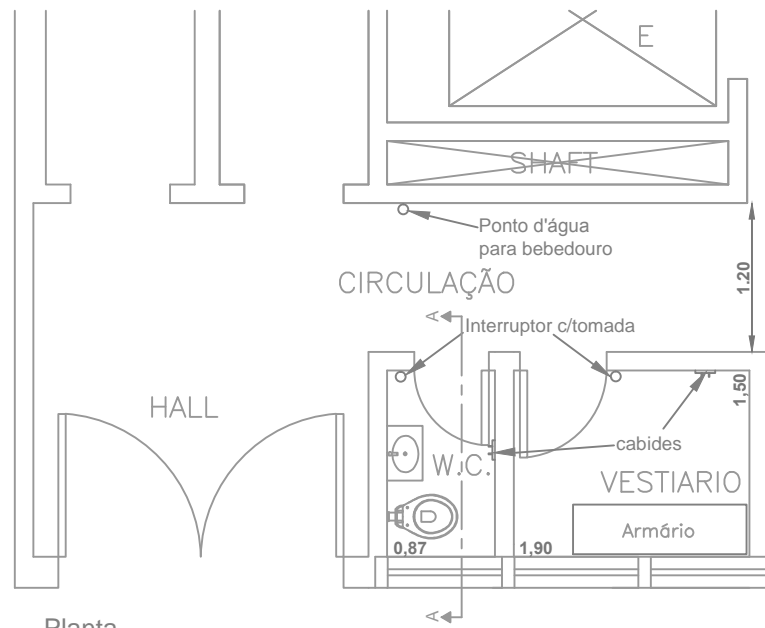
Planta
