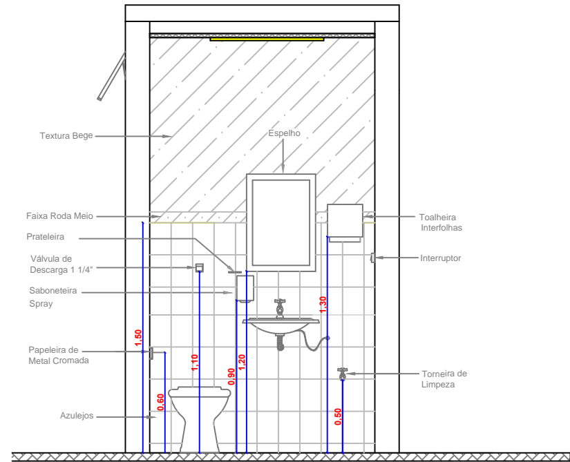
Corte AA
