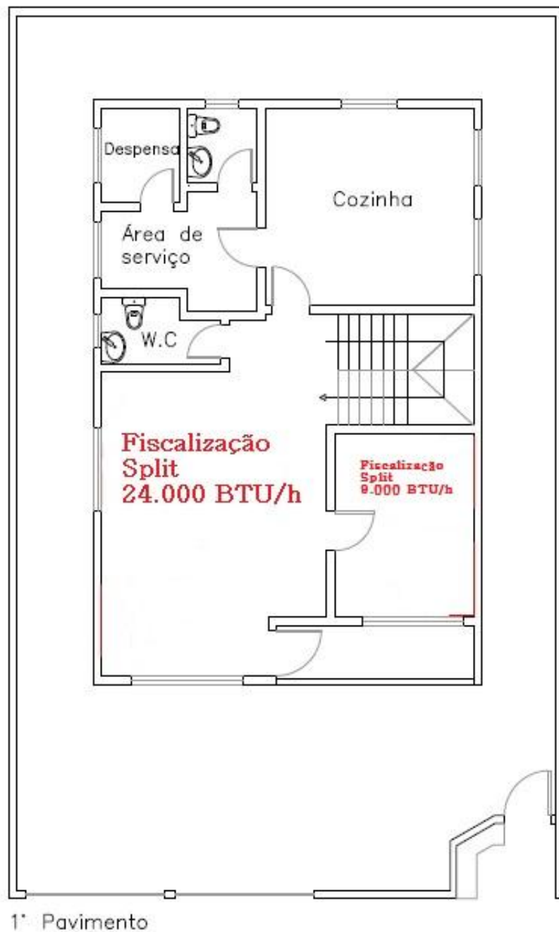
Figura nº 6 – Ar-condicionado 1º pavimento
