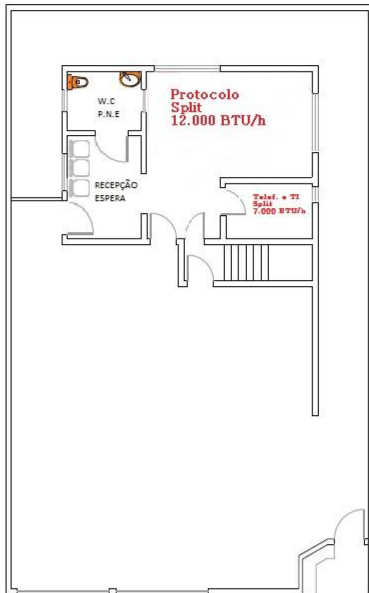
Figura nº 7 – Ar-condicionado pavimento térreo
