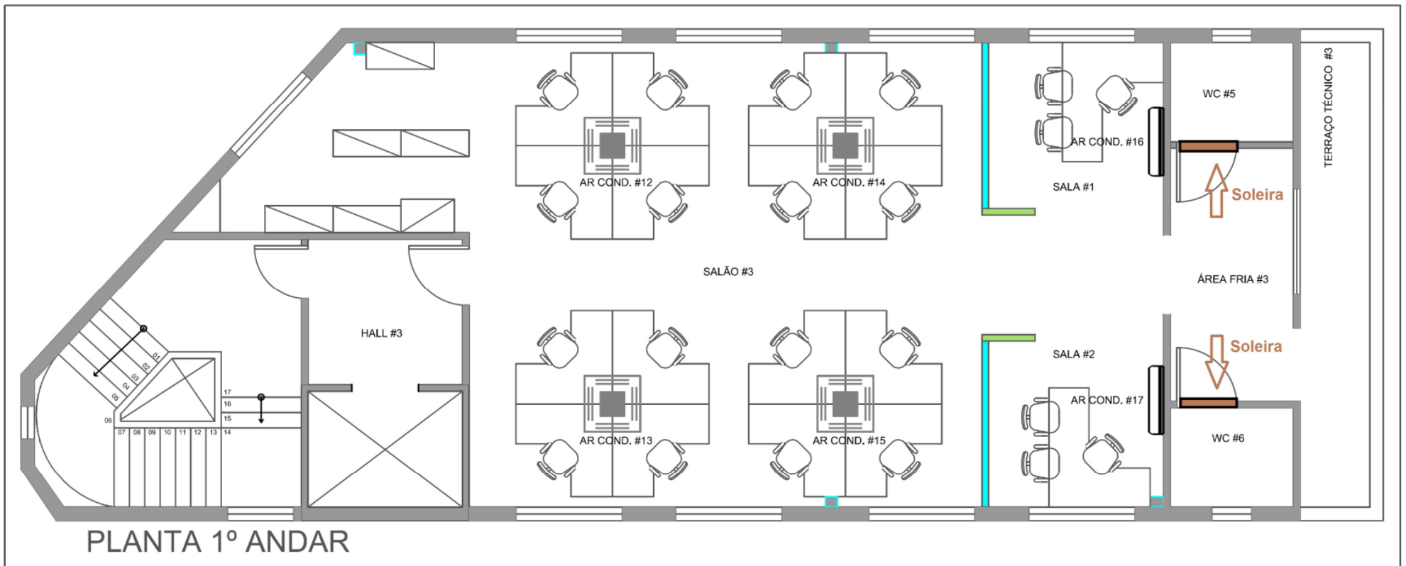
PLANTA PAVIMENTO TIPO 1
