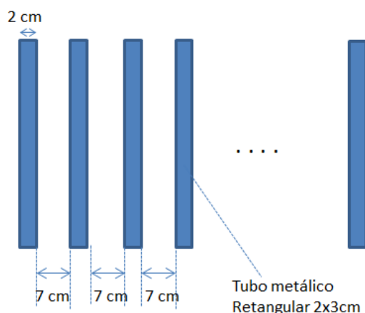
Figura 2 – Padrão dos painéis do fechamento – tubos 2x3 cm verticais.
