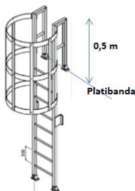
Figura 3 – Ilustrativo da escada tipo marinheiro.
