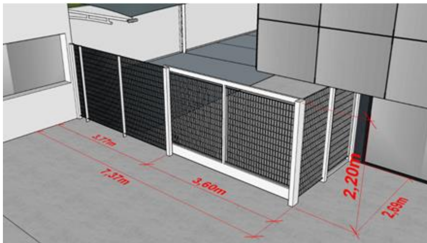
Figura 1 – Identificação e dimensões dos fechamentos.
