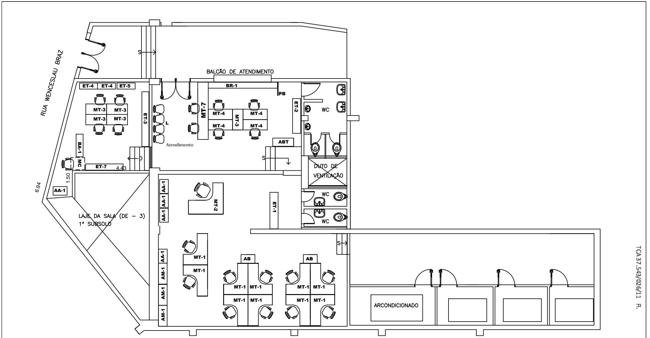
PLANTA – TÉRREO
