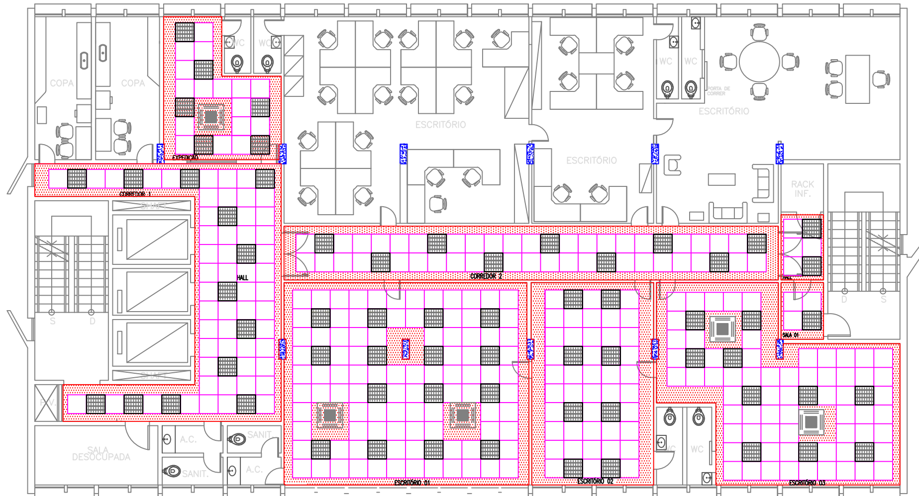
PLANTA DO 3º PAVIMENTO – ANEXO I
