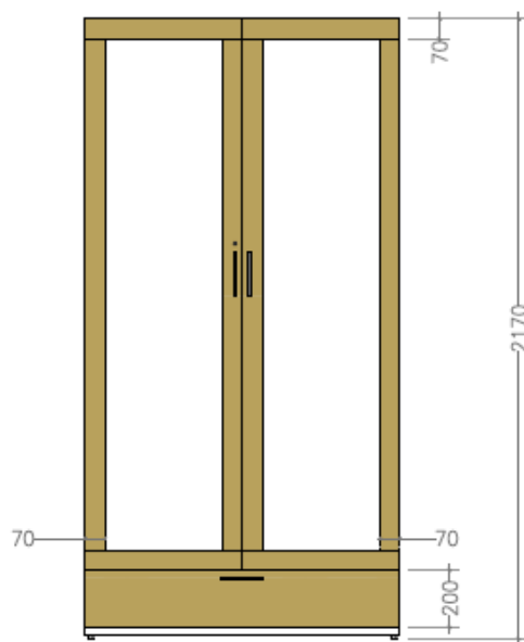
Elevação
