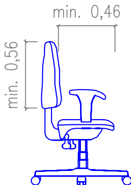
Elevação Lateral
