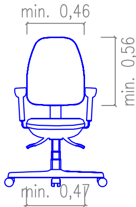
Elevação Frontal
