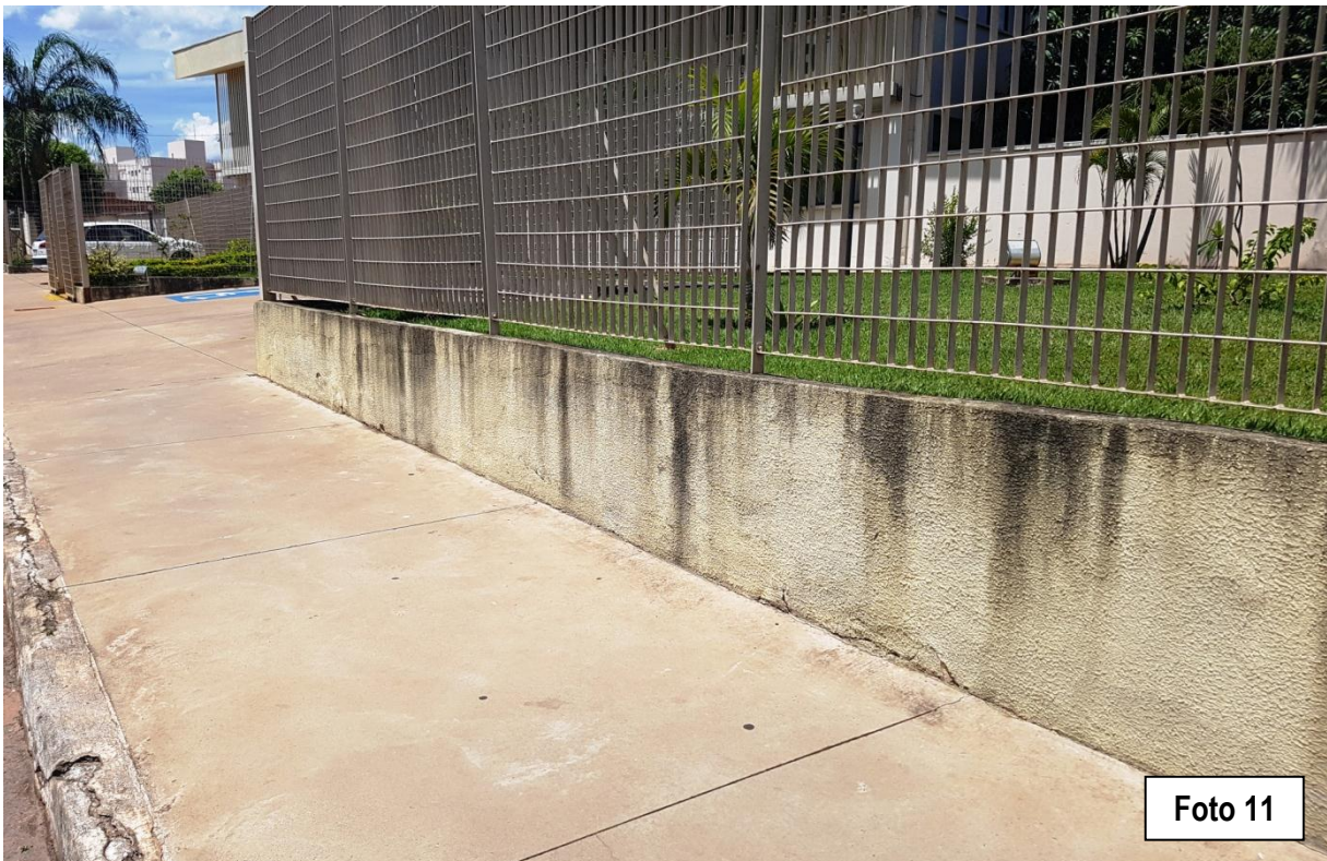
Fachada com parte do reboco deteriorado e pintura desgastada
