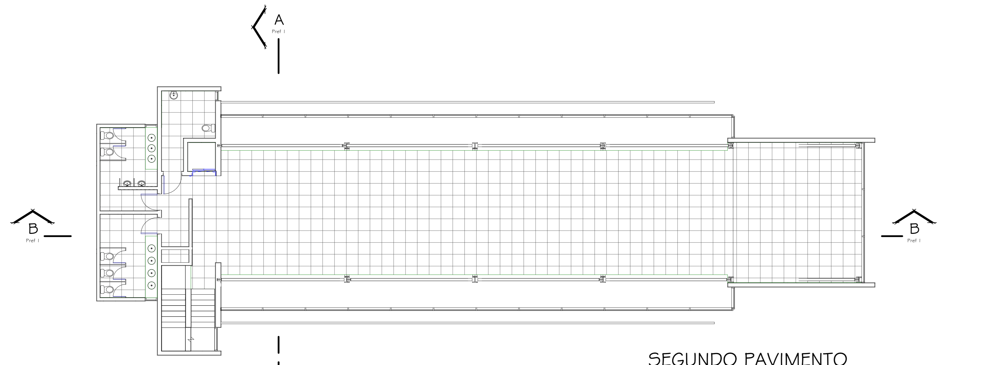
SEGUNDO PAVIMENTO
