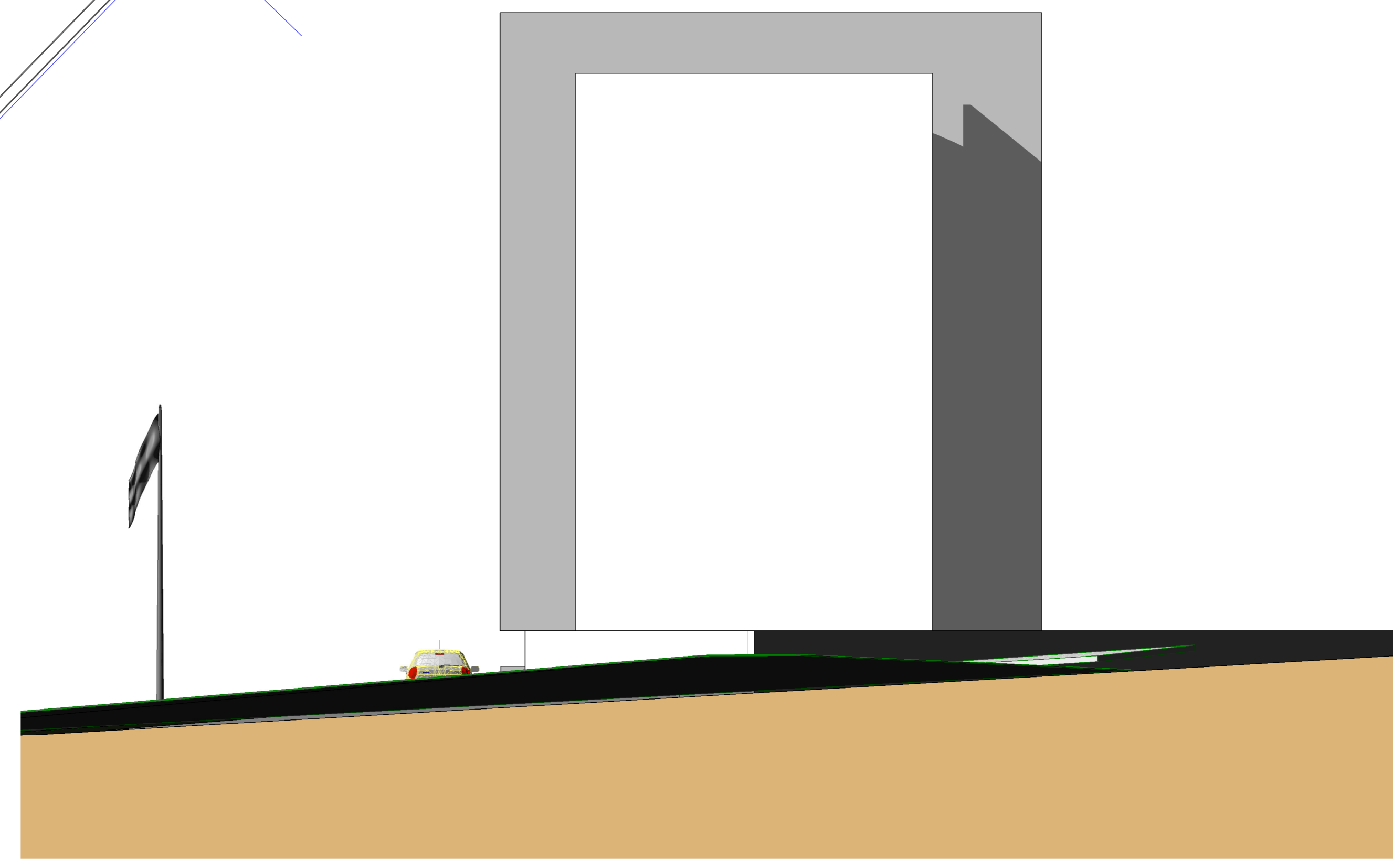
ELEVAÇÃO NORTE 1/100
