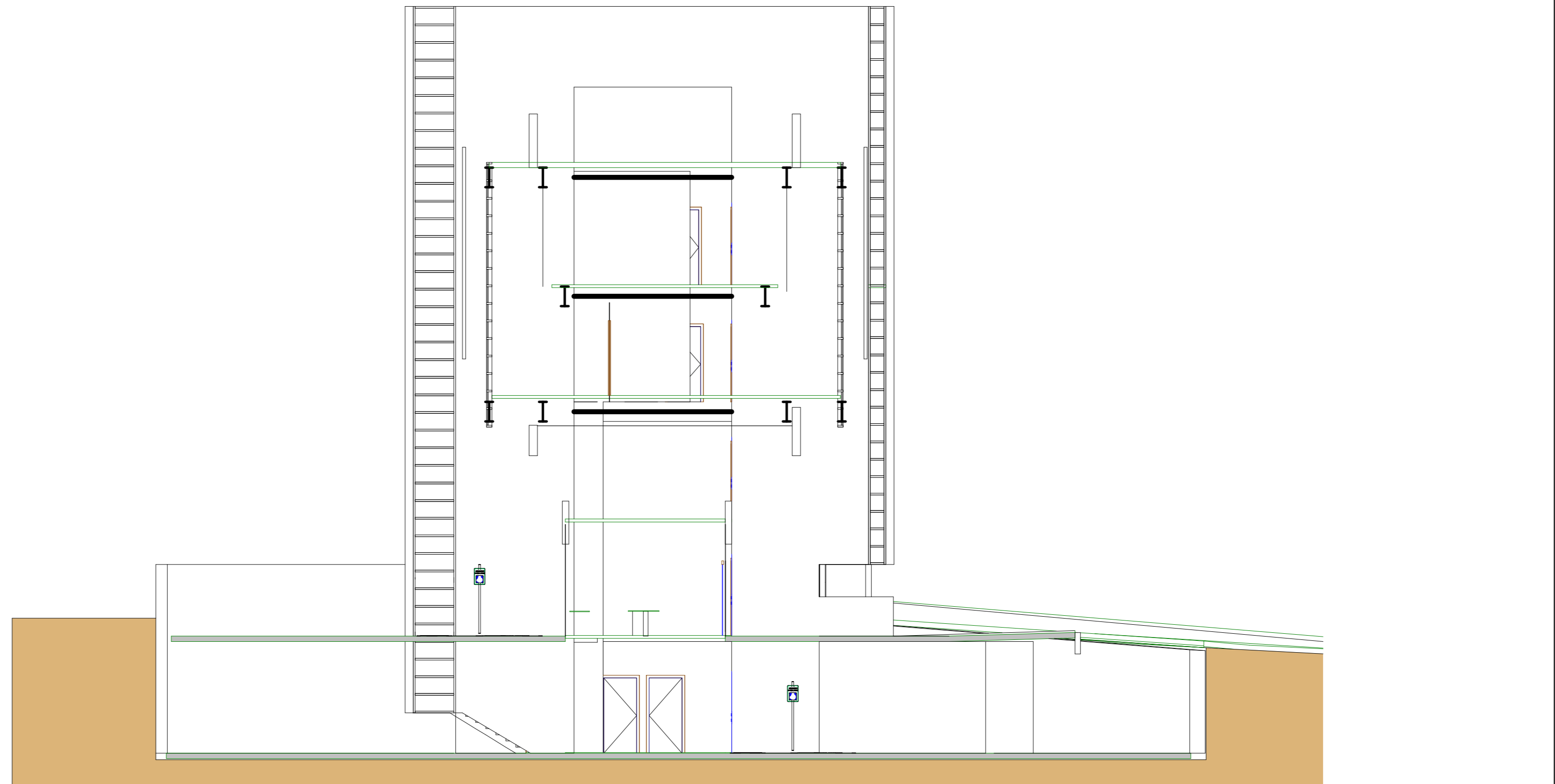
CORTE AA
