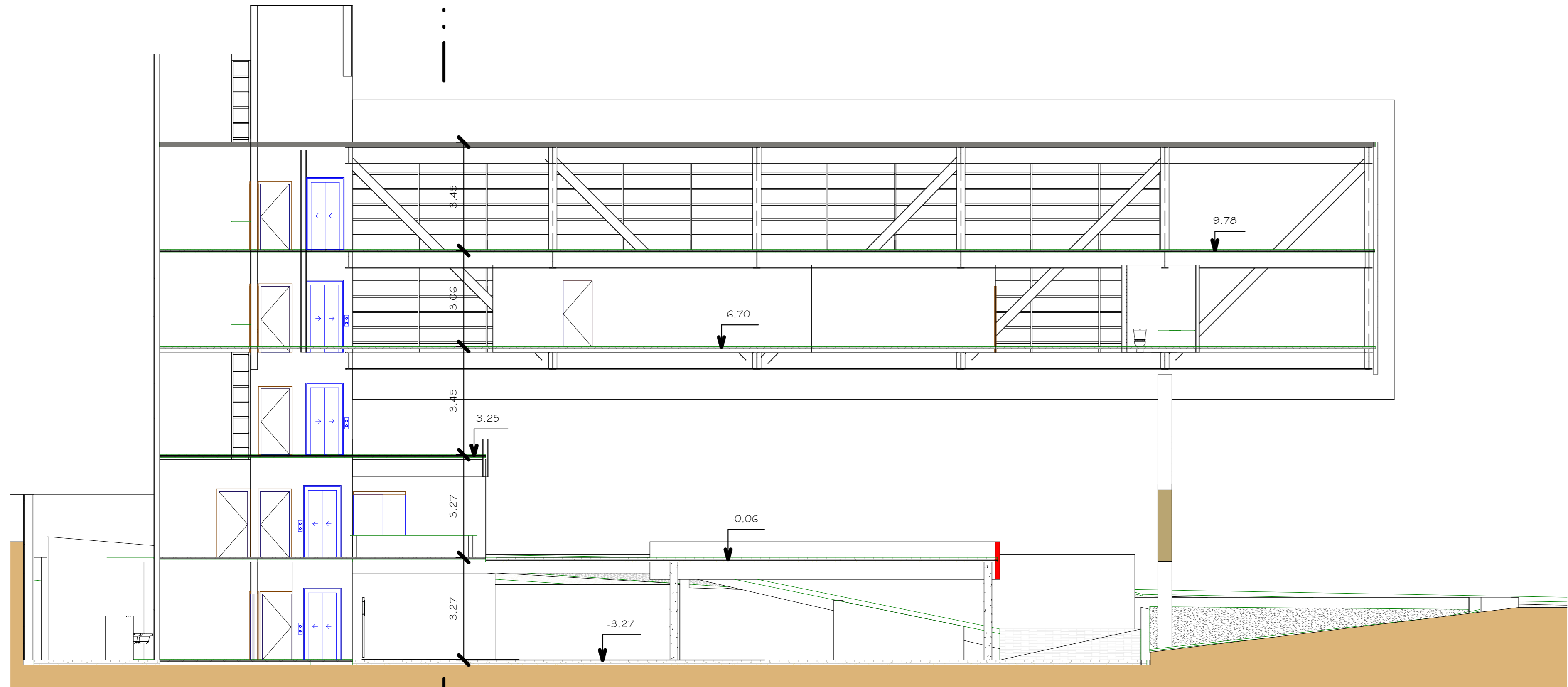
CORTE BB
