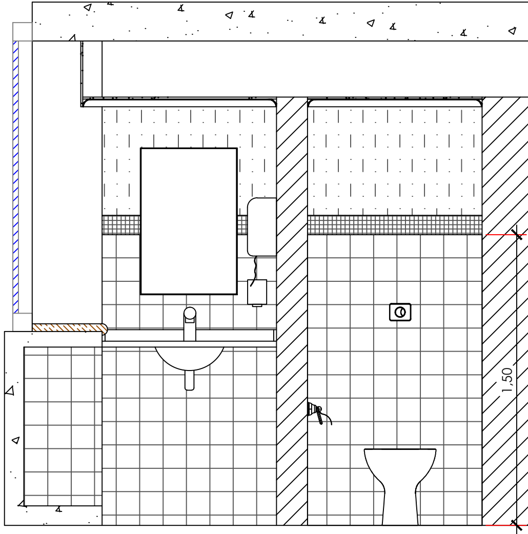
CORTE AA
