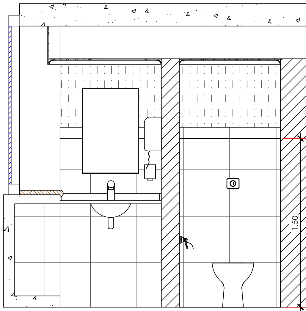
CORTE AA
