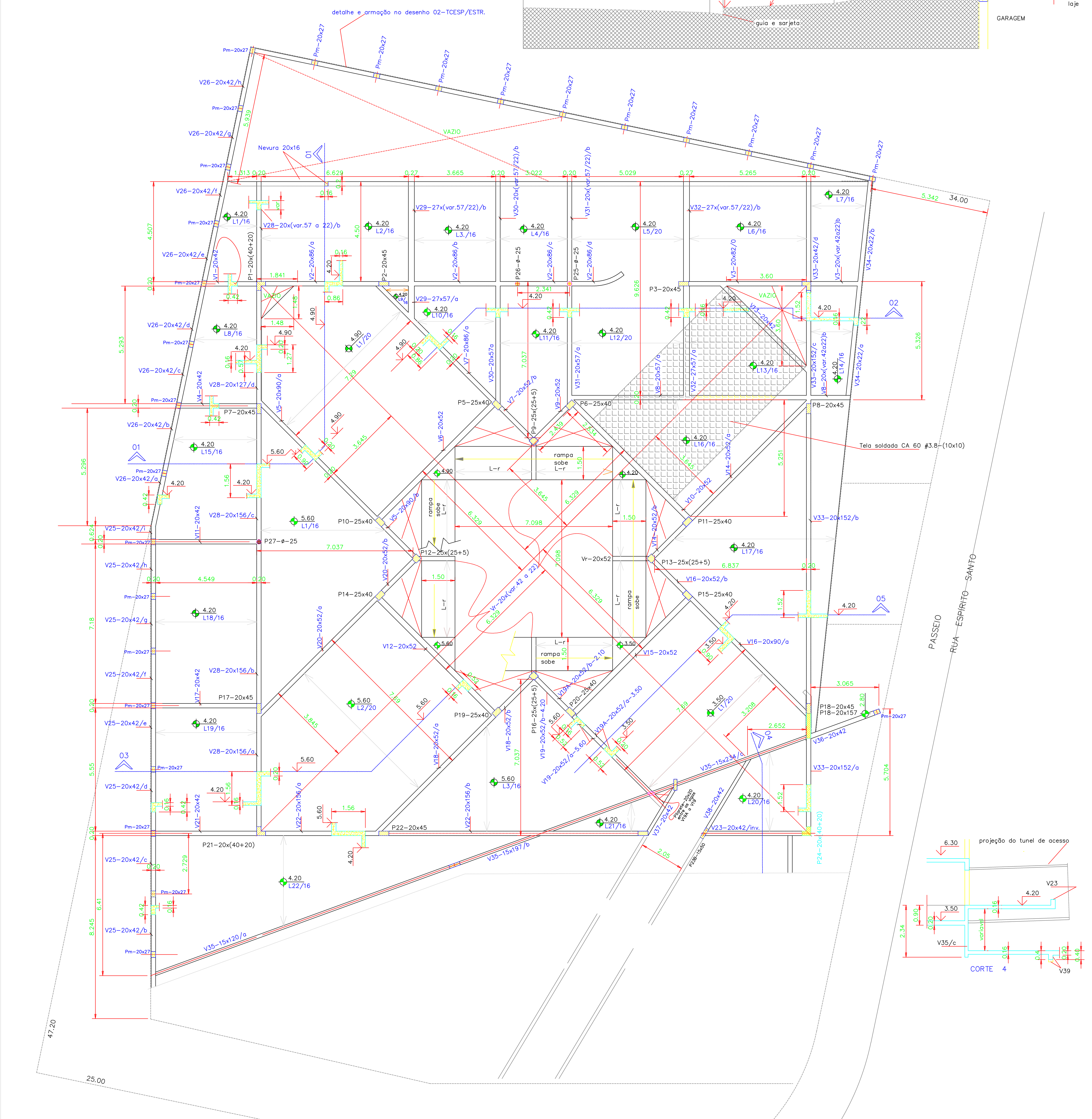
Planta de forma das lajes nível Terreno ESCALA 1:75
