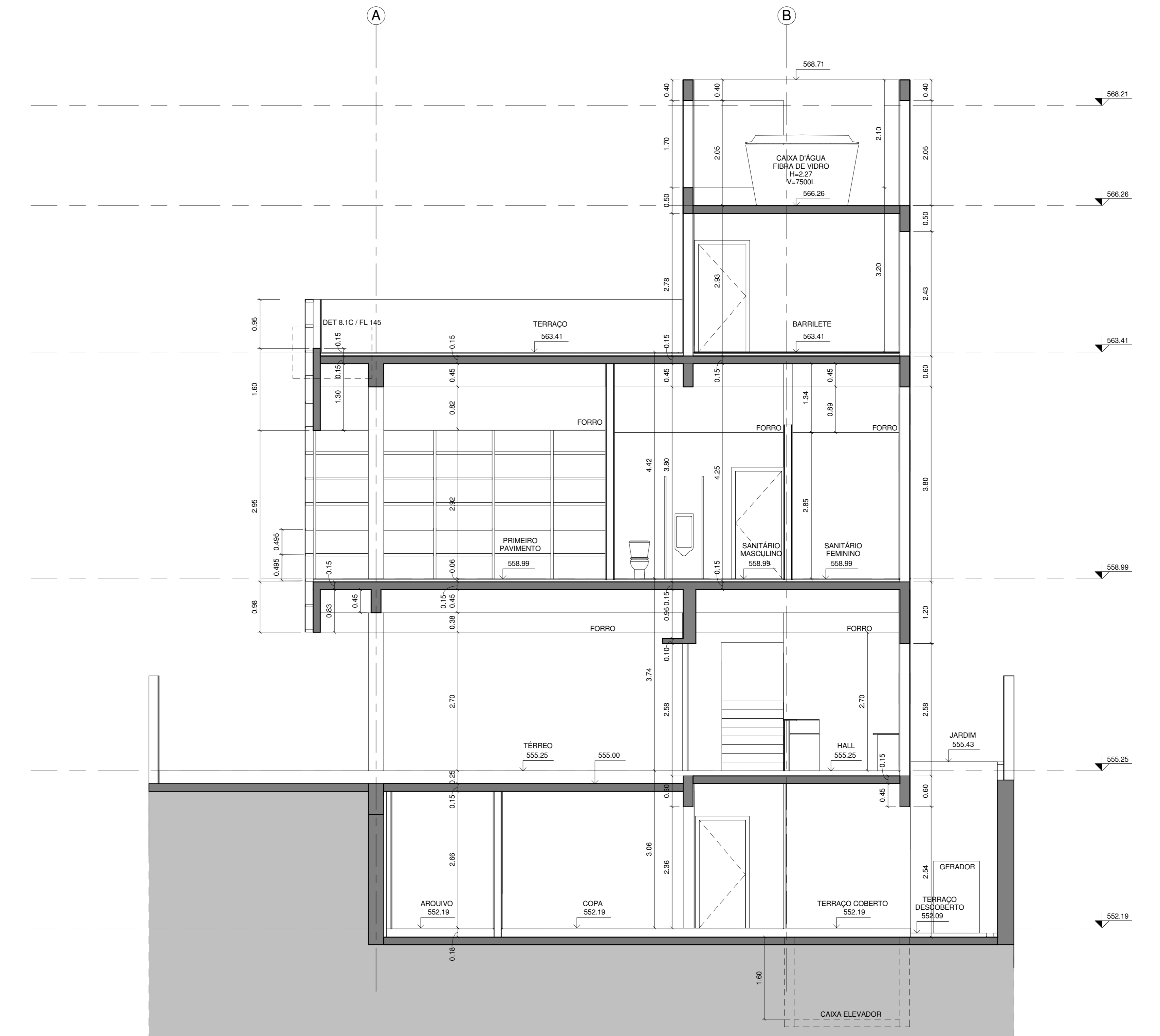
CORTE B-B 1 : 50
