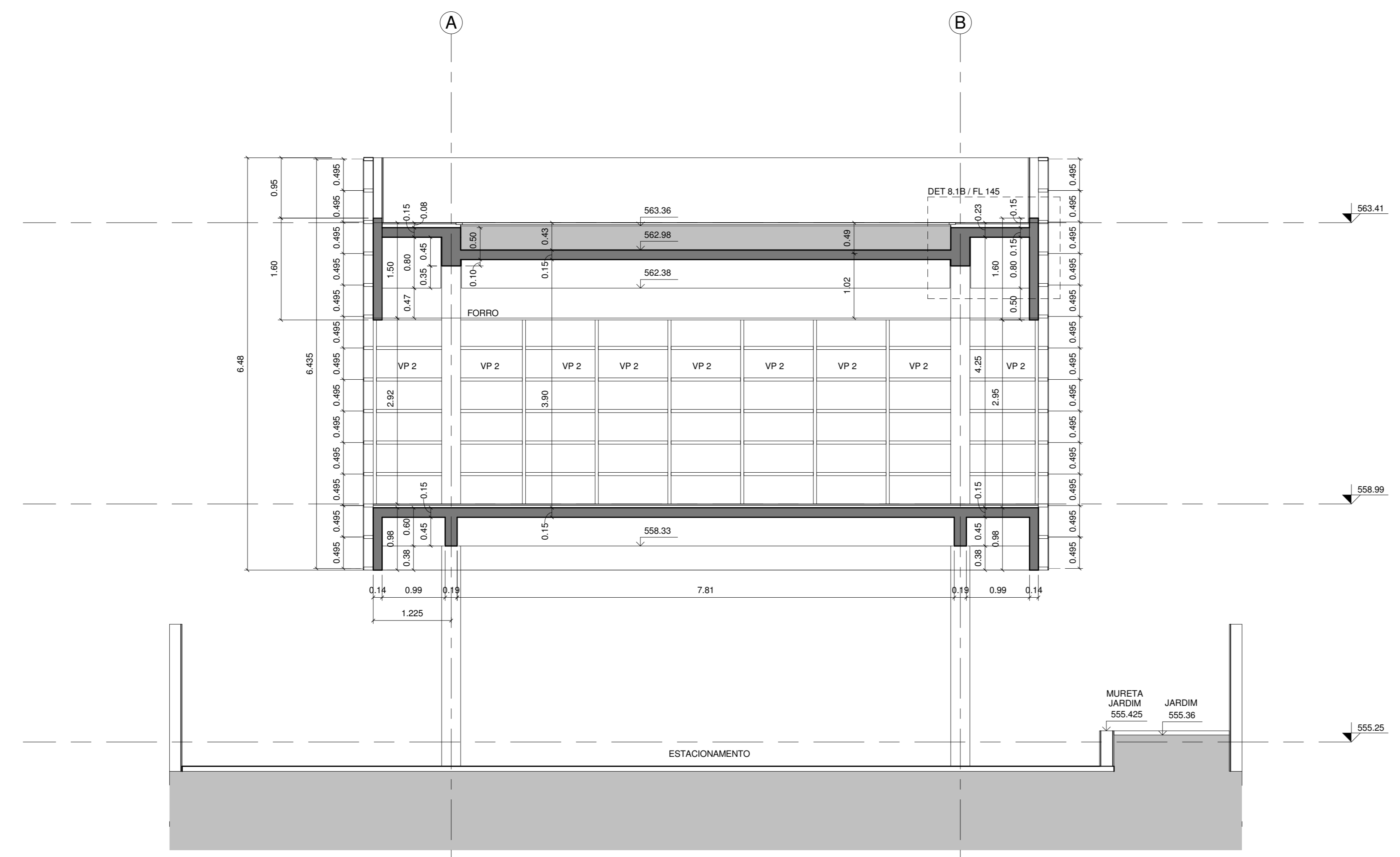
CORTE A-A 1 : 50
