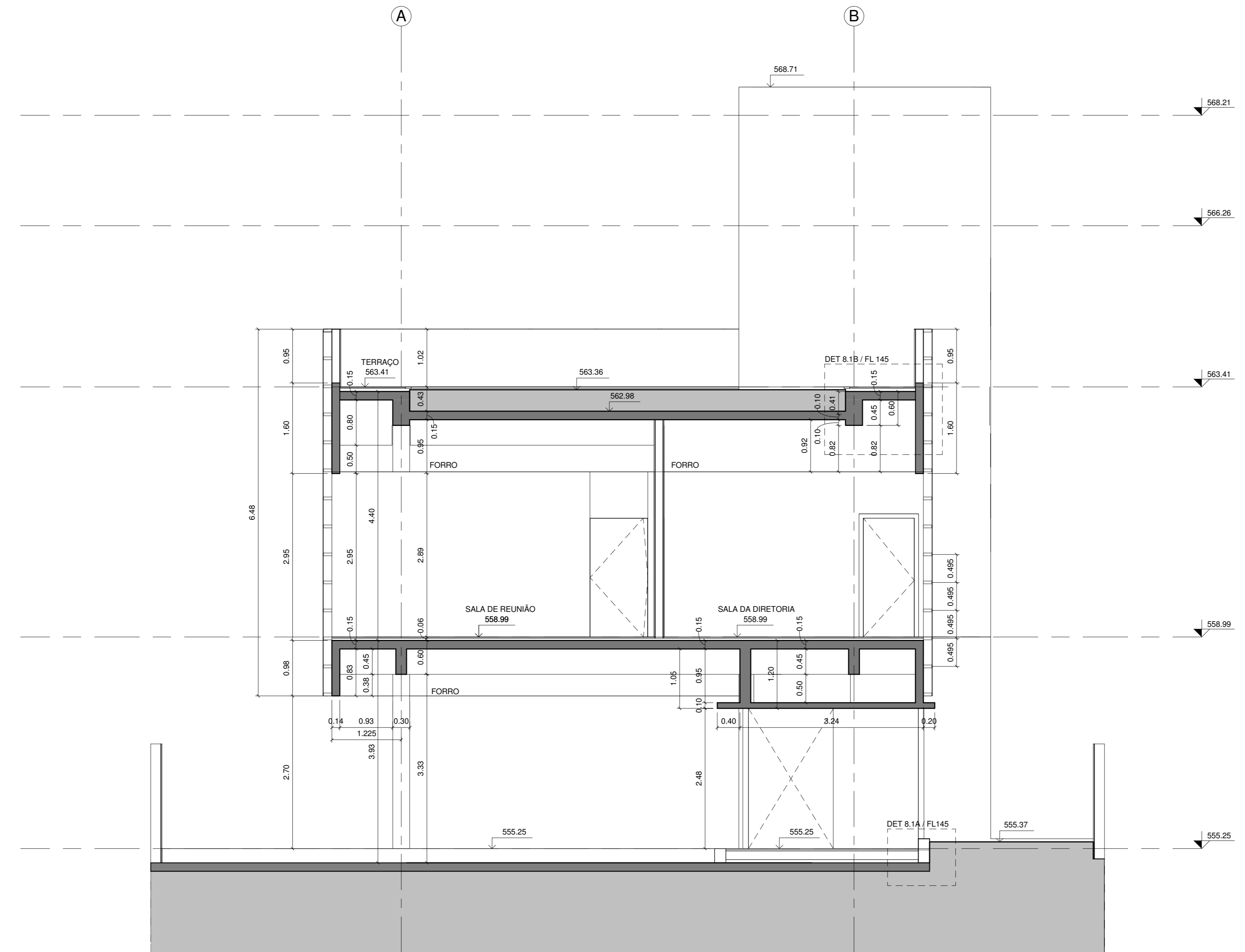
CORTE C-C 1 : 50
