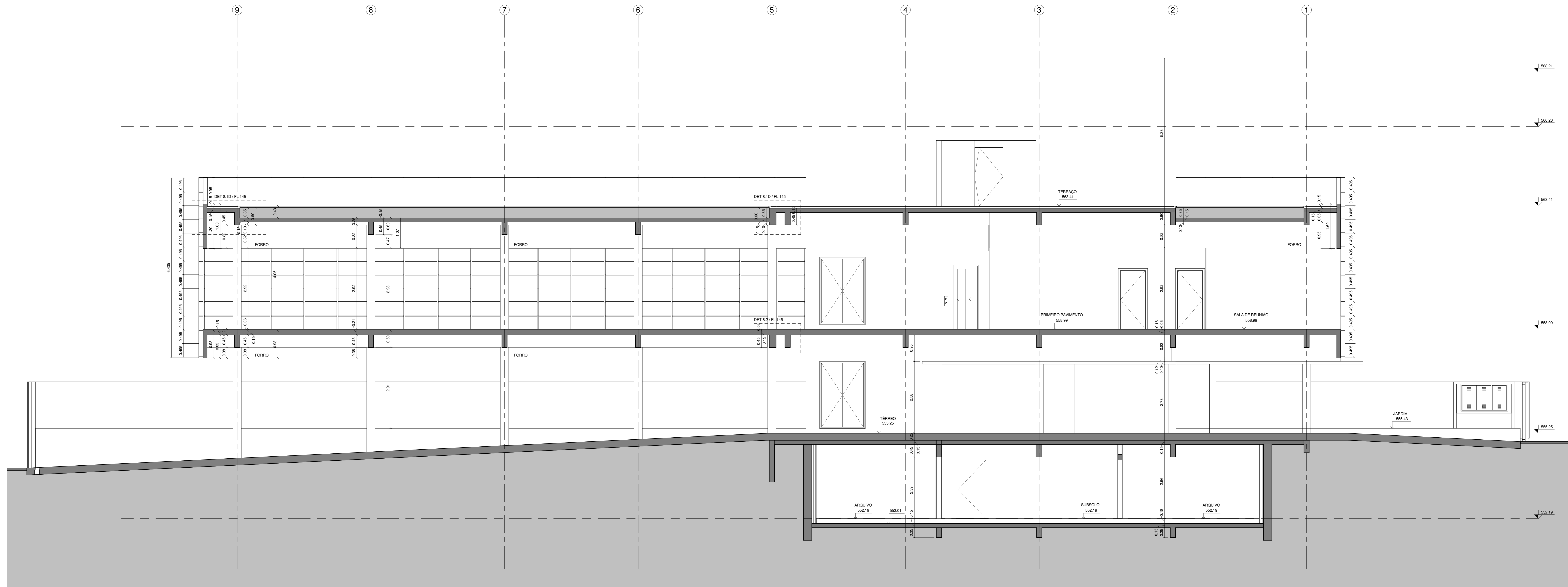
CORTE D-D 1 : 50
