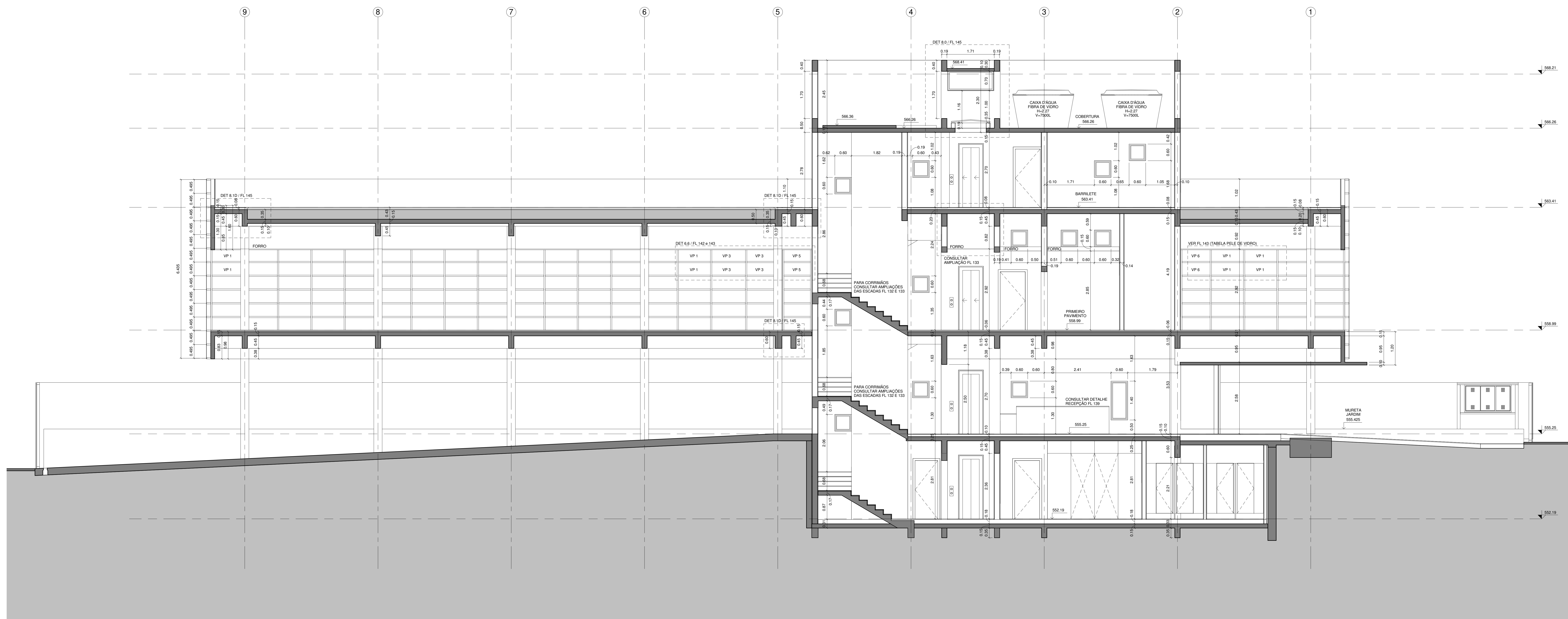
CORTE E-E 1:50
