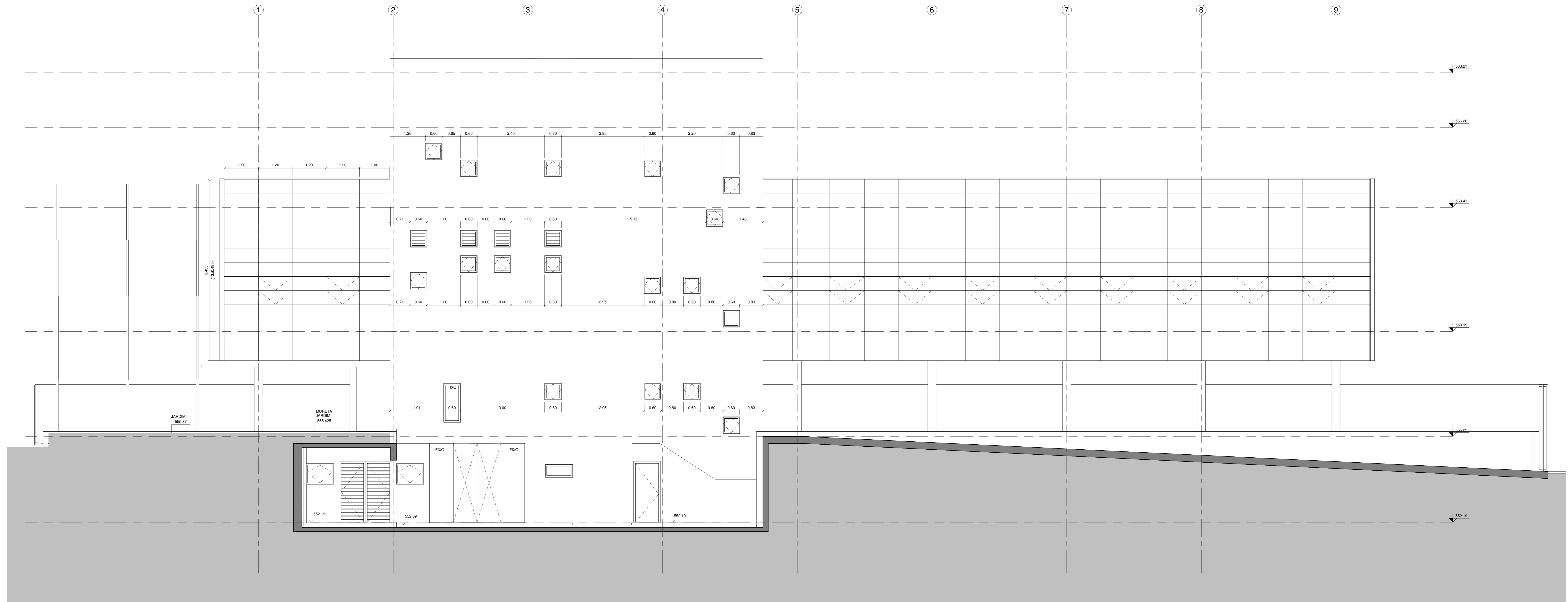
ELEVAÇÃO 1 1 : 50
