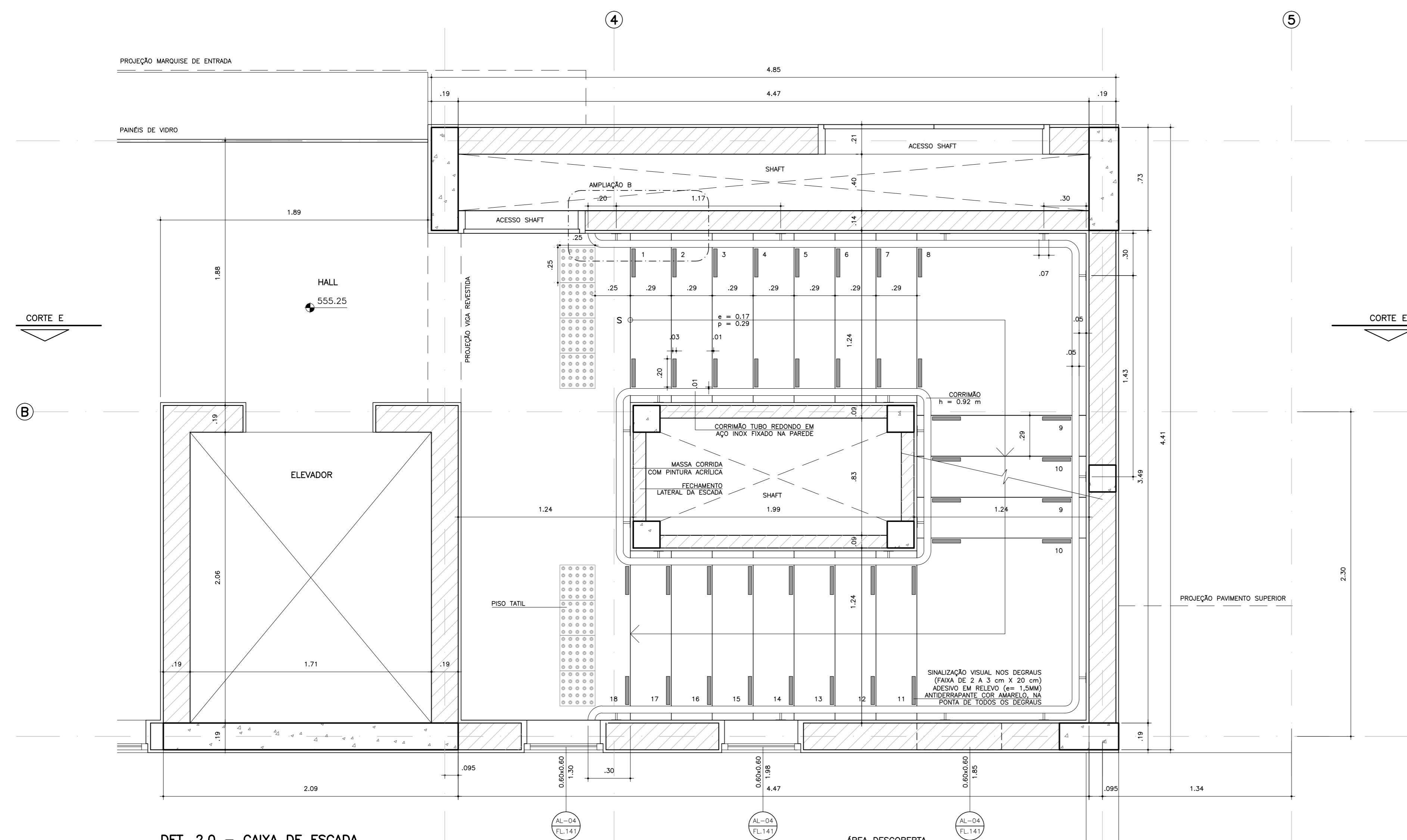
DET. 2.0 - CAIXA DE ESCADA PLANTA TÉRREO ESC 1:20
