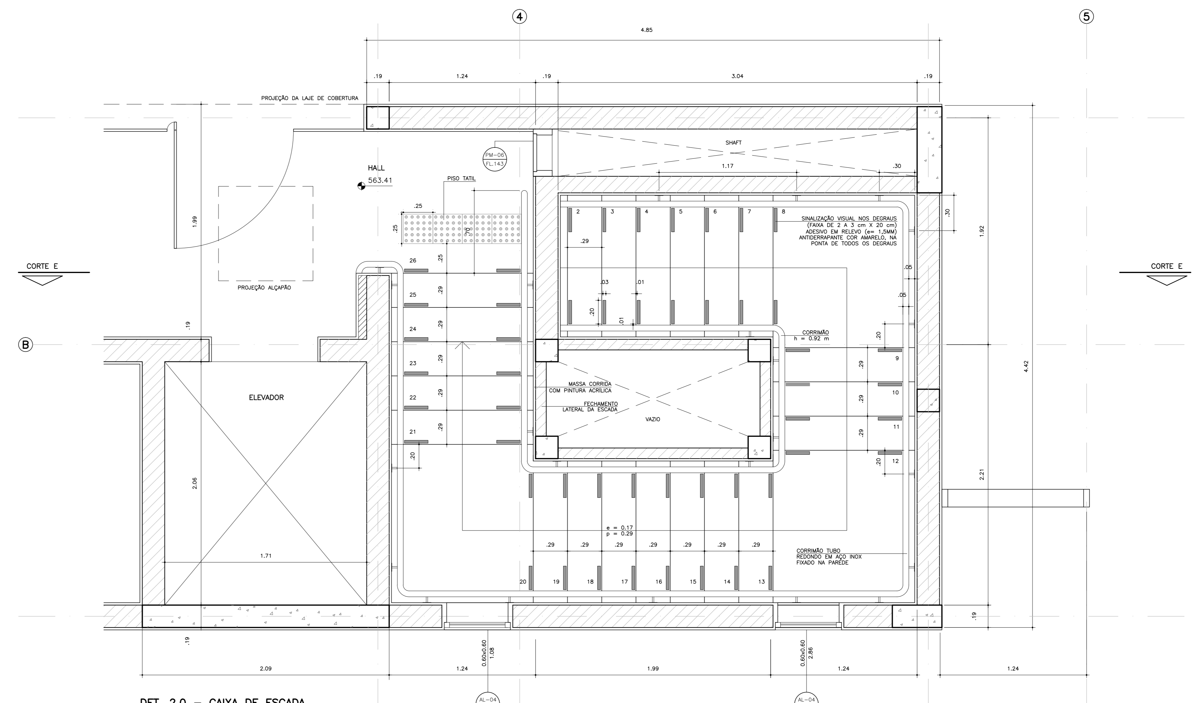
DET. 2.0 - CAIXA DE ESCADA PLANTA COBERTURA ESC 1:20
