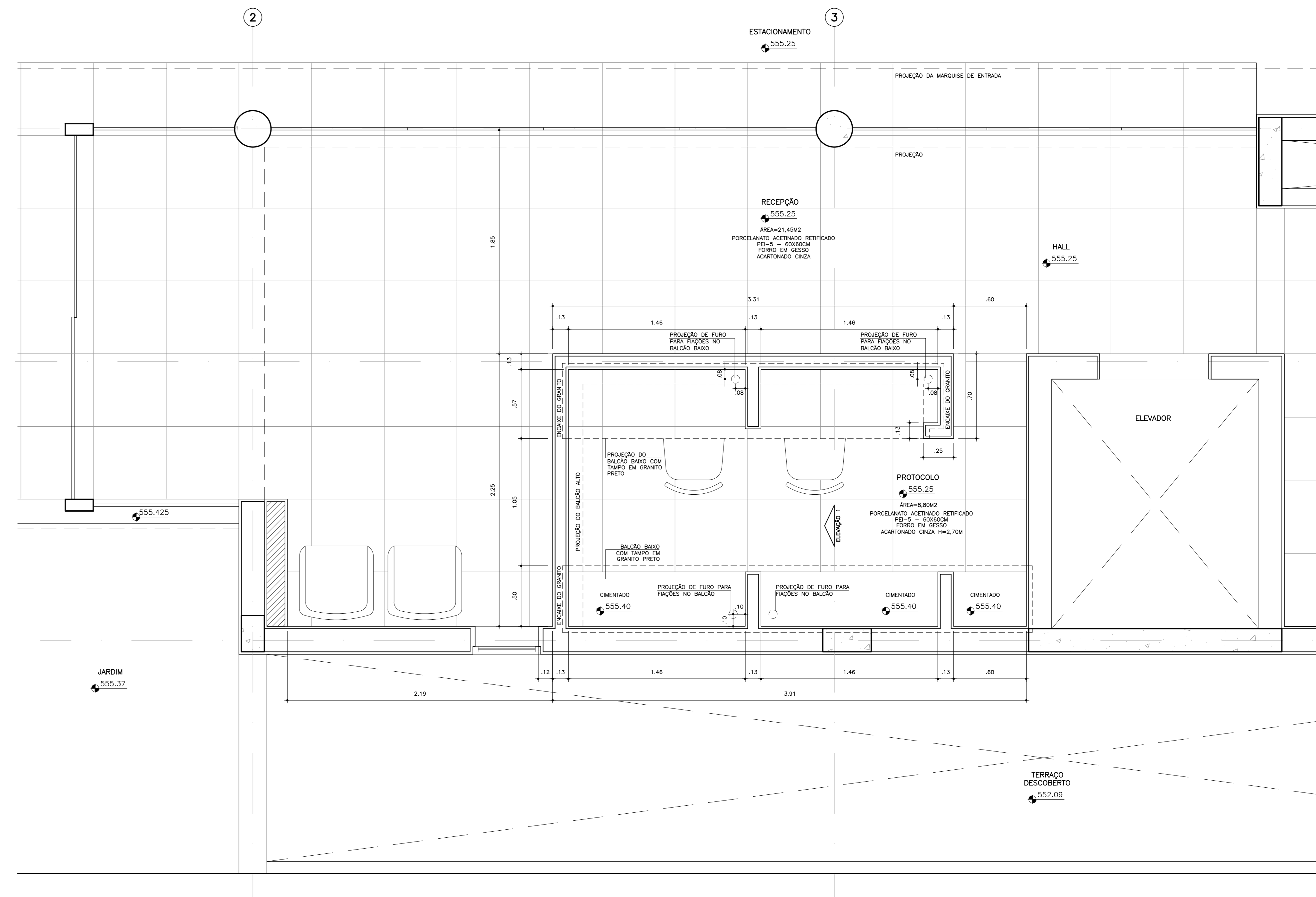
DET. 4.0 - AMPLIAÇÃO DA RECEPÇÃO/PROTOCOLO PLANTA ALVENARIA DE APOIO DO BALCÃO ESC. 1:20
