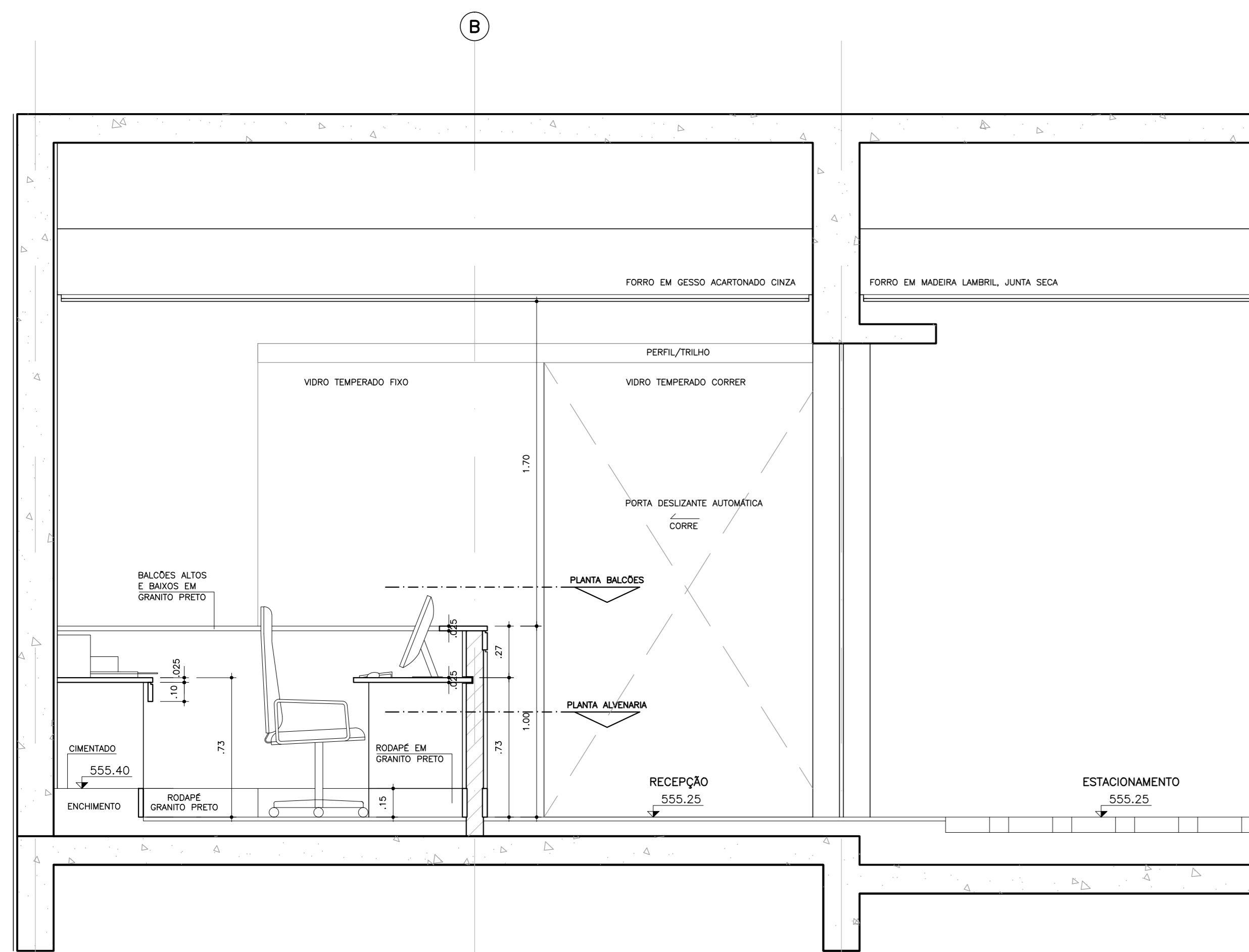
DET. 4.0 - AMPLIAÇÃO DA RECEPÇÃO/PROTOCOLO ELEVACÃO 1 ESC. 1:20
