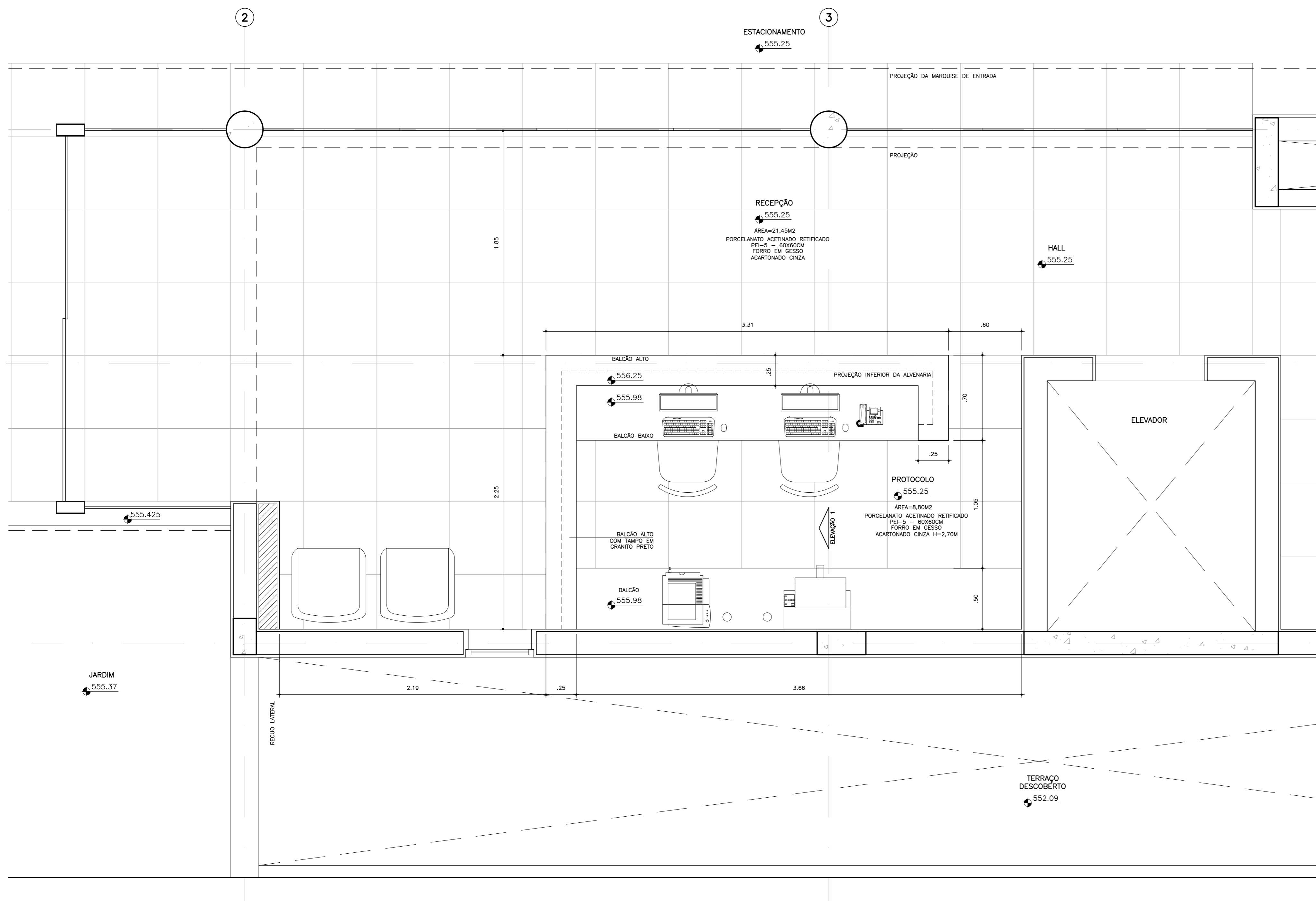
DET. 4.0 - AMPLIAÇÃO DA RECEPÇÃO/PROTOCOLO PLANTA BALCÕES ESC. 1:20
