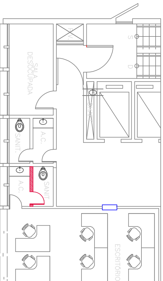
Planta 3º andar - Anexo I
